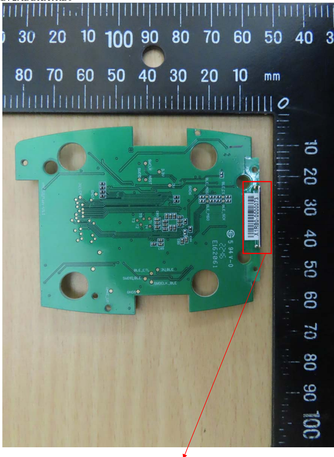
Rod antenna
