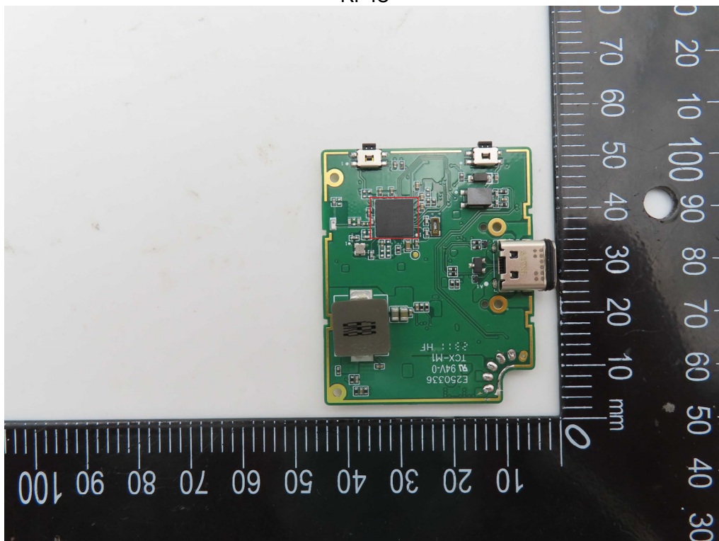
RF IC
