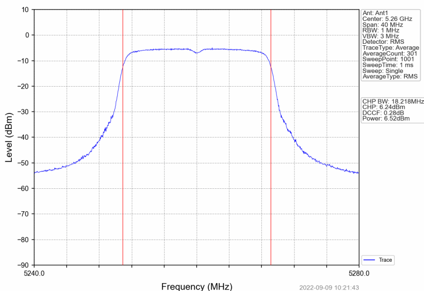
802.11n(HT20)_LCH_5260MHz_Ant1_NTNV
