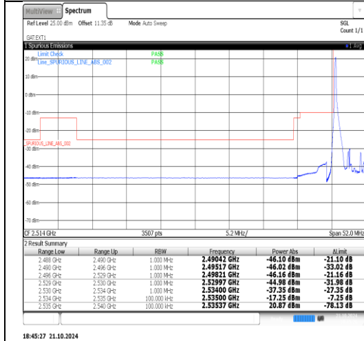
41(2535-2655)-5MHz-QPSK-40065-1RB#24-PASS
