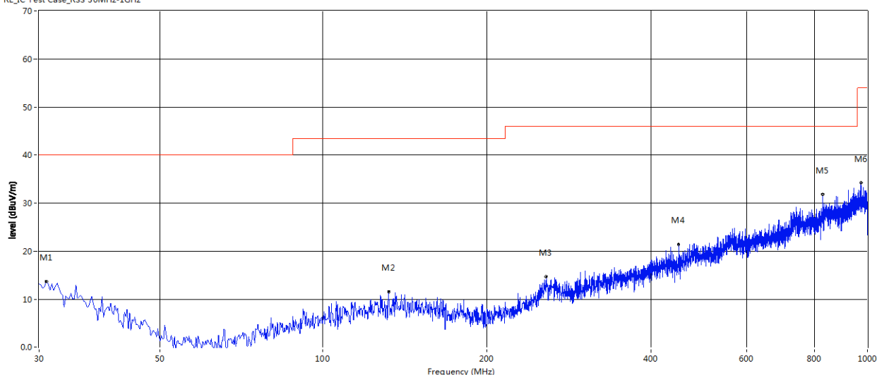
RE_IC Test Case_RSS 30MHz-1GHz
