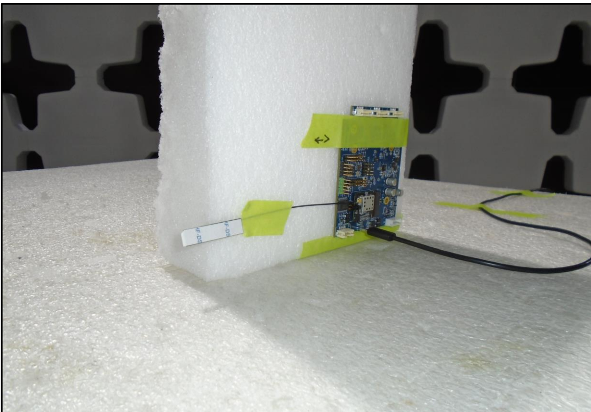
PCB ant (2)
