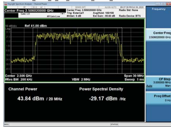
Ch_Power_TM1_1_1C_20MBW_2506_TX4
