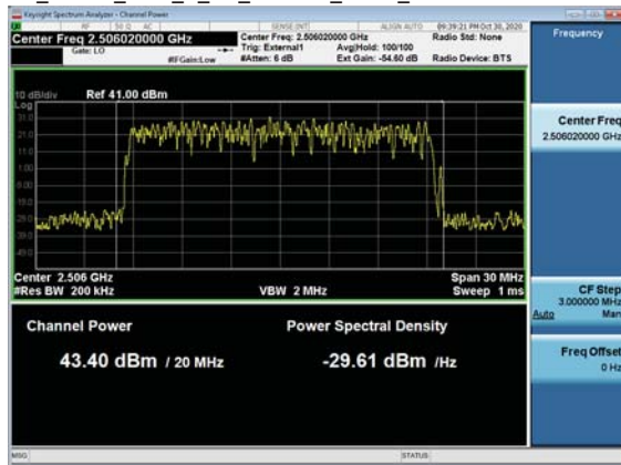
Ch_Power_TM1_1_1C_20MBW_2506_TX3
