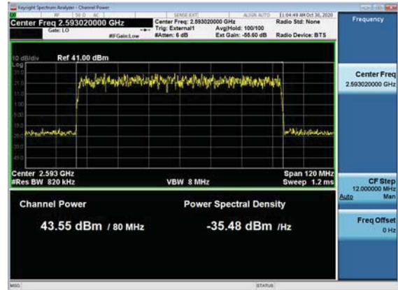
Ch_Power_TM1_1_1C_80MBW_2593_TX4
