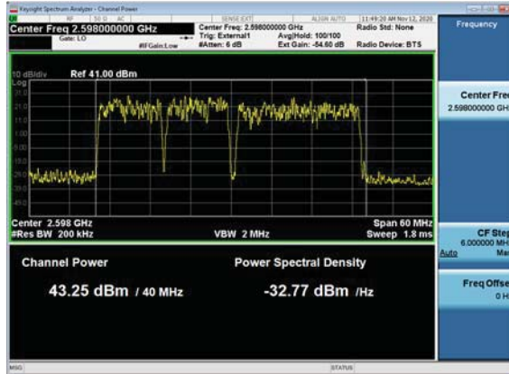
Ch_Power_TM1_1_3C_10+10+20MBW _2583_2593_2608_TX3 QPSK 16QAM 256QAM
