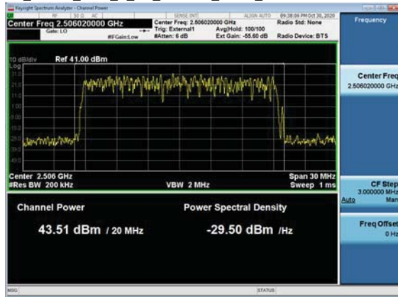
Ch_Power_TM1_1_1C_20MBW_2506_TX1
