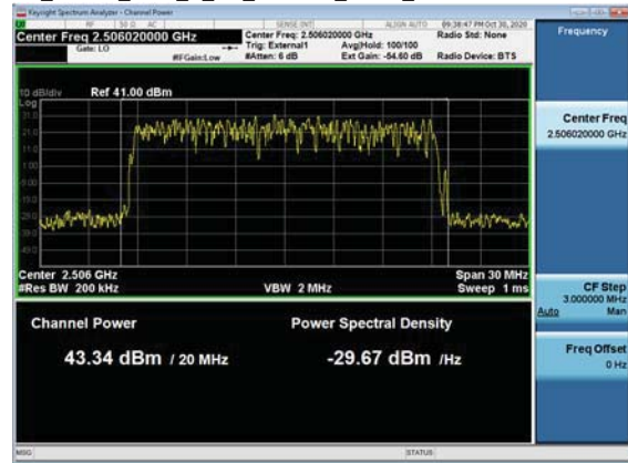
Ch_Power_TM1_1_1C_20MBW_2506_TX2
