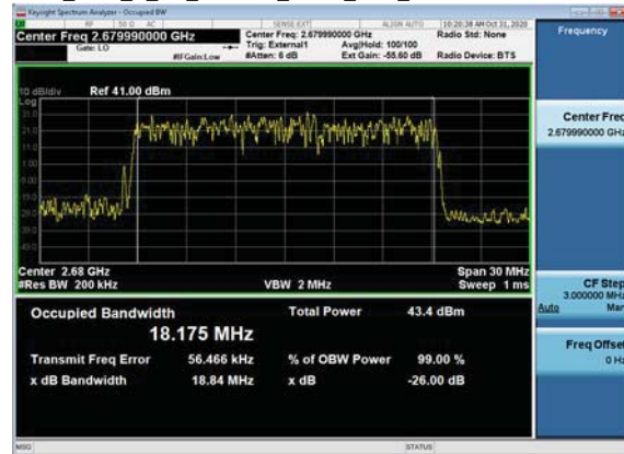
OBW_TM1_1_1C_20MBW_2679_TX4_2679
