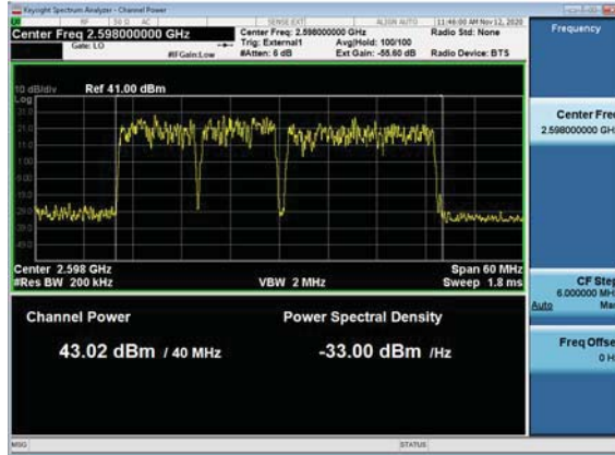
Ch_Power_TM1_1_3C_10+10+20MBW _2583_2593_2608_TX1 QPSK 16QAM 256QAM
