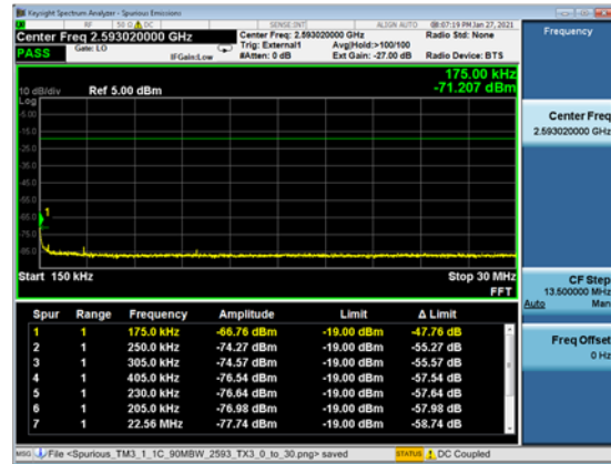
150kHz – 30MHz
