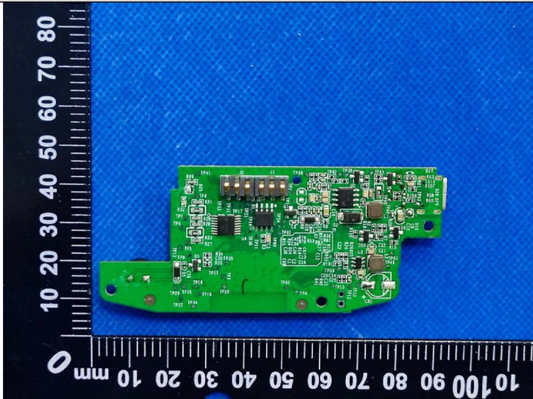
EUT Photo
