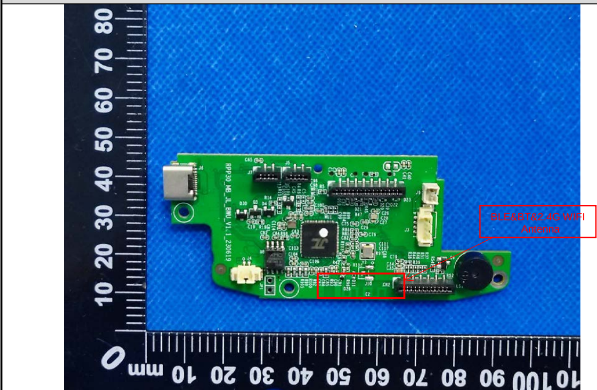
EUT Photo
