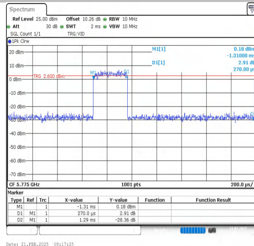
NTNV-11AX80SISO-Ant1-5775
