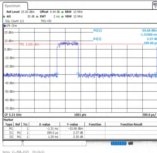
NTNV-11AX80SISO-Ant1-5210
