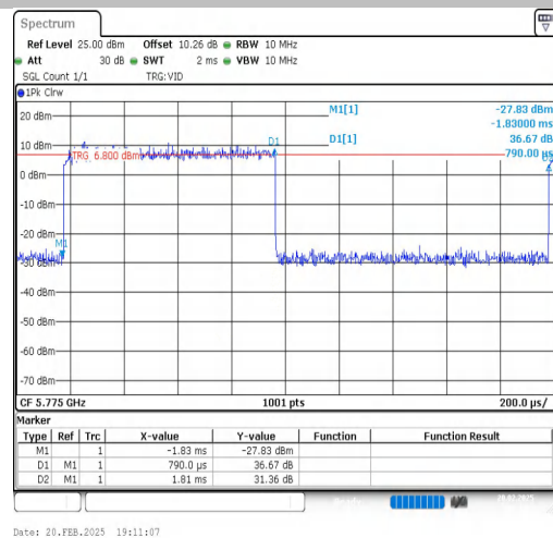
NTNV-11AC80SISO-Ant1-5775
