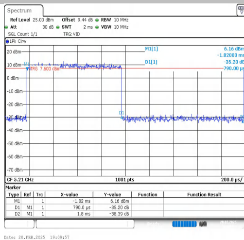
NTNV-11AC80SISO-Ant1-5210
