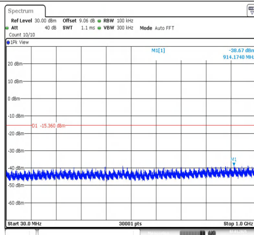
BLE_2M-Ant1-2440-30~1000-PASS
