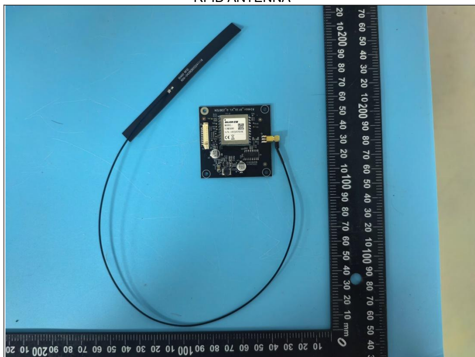
RFID ANTENNA
