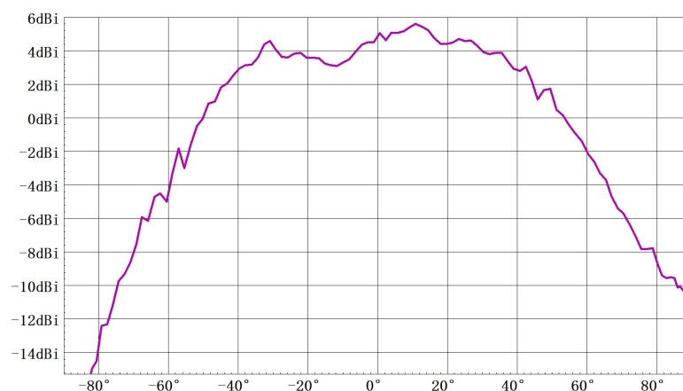
方位面方向图 (TX1) Freq:60.0GHz
