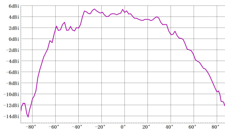
方位面方向图 (TX0) Freq:59.0GHz
