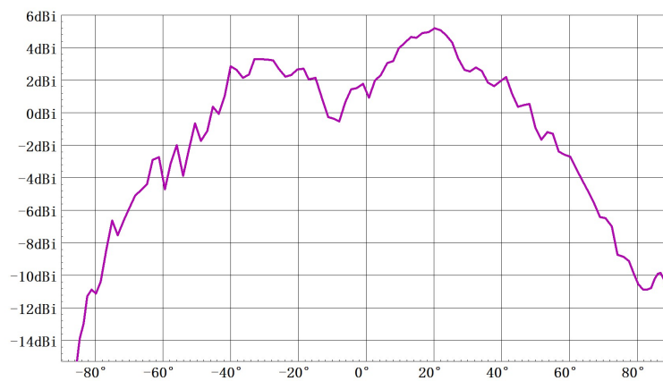
方位面方向图 (TX0) Freq:62.0GHz
