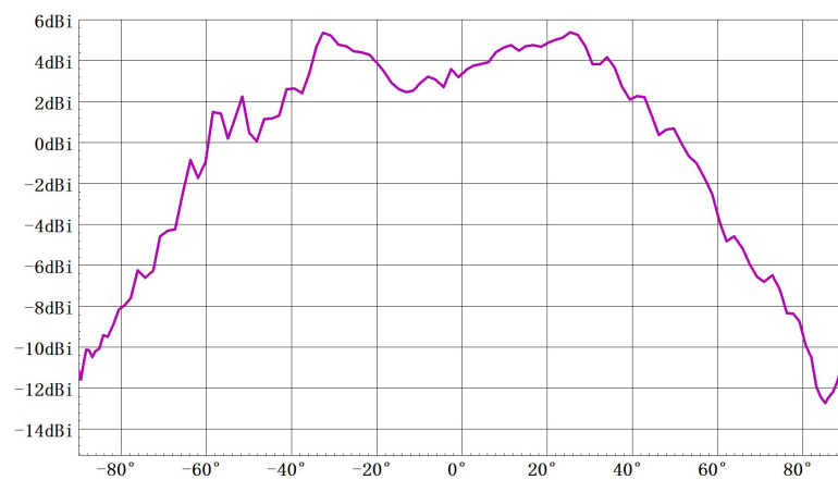
方位面方向图 (TX0) Freq:61.0GHz
