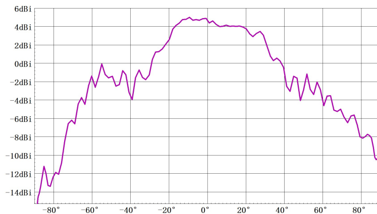
方位面方向图 (TX1) Freq:57.0GHz
