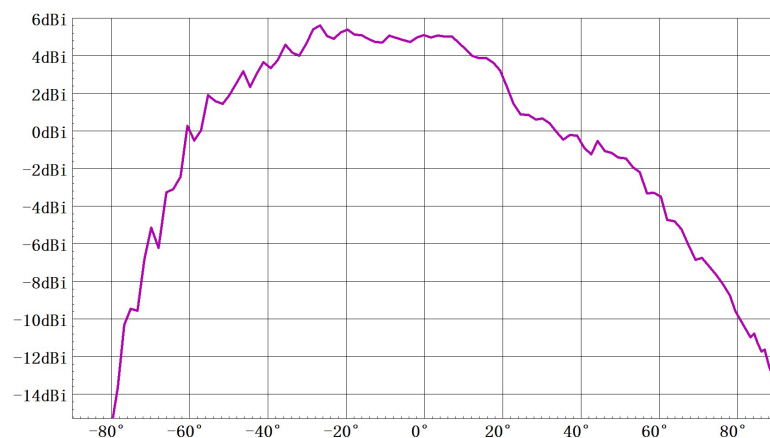
方位面方向图 (TX0) Freq:60.0GHz
