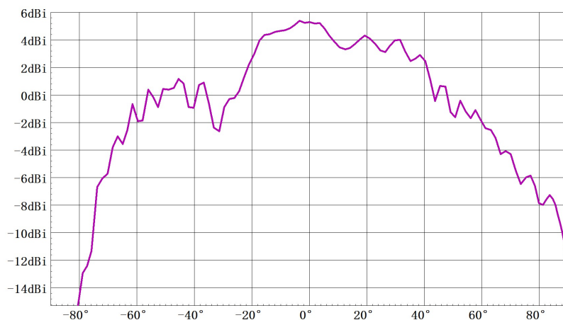
方位面方向图 (TX1) Freq:61.0GHz
