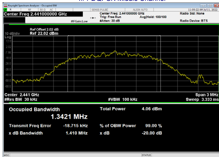
\pi/4 -DQPSK Middle Channel
