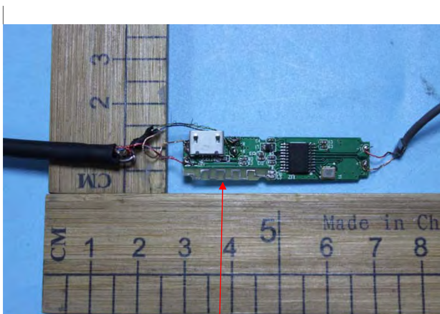
Antenna
