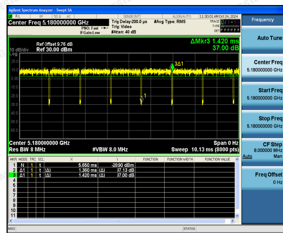
802.11a
