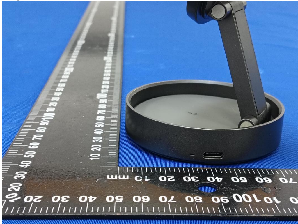
8) EUT Photo
