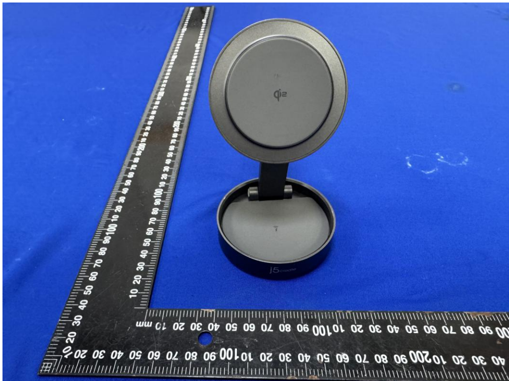
2) EUT Photo
