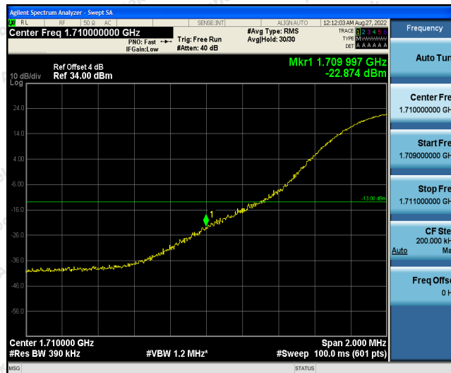
Band4-20MHz-QPSK-20050-1RB#99
