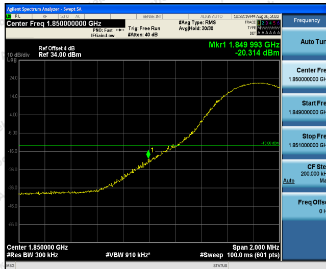
Band2-15MHz-QPSK-18675-1RB#74
