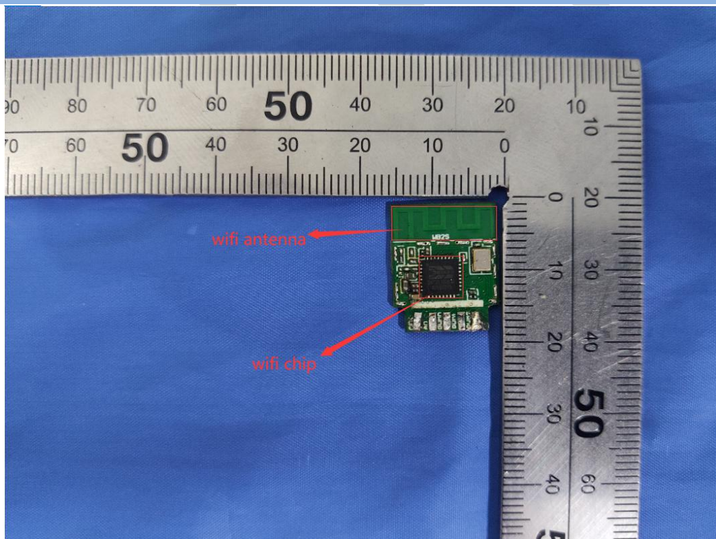
WI-FI module
