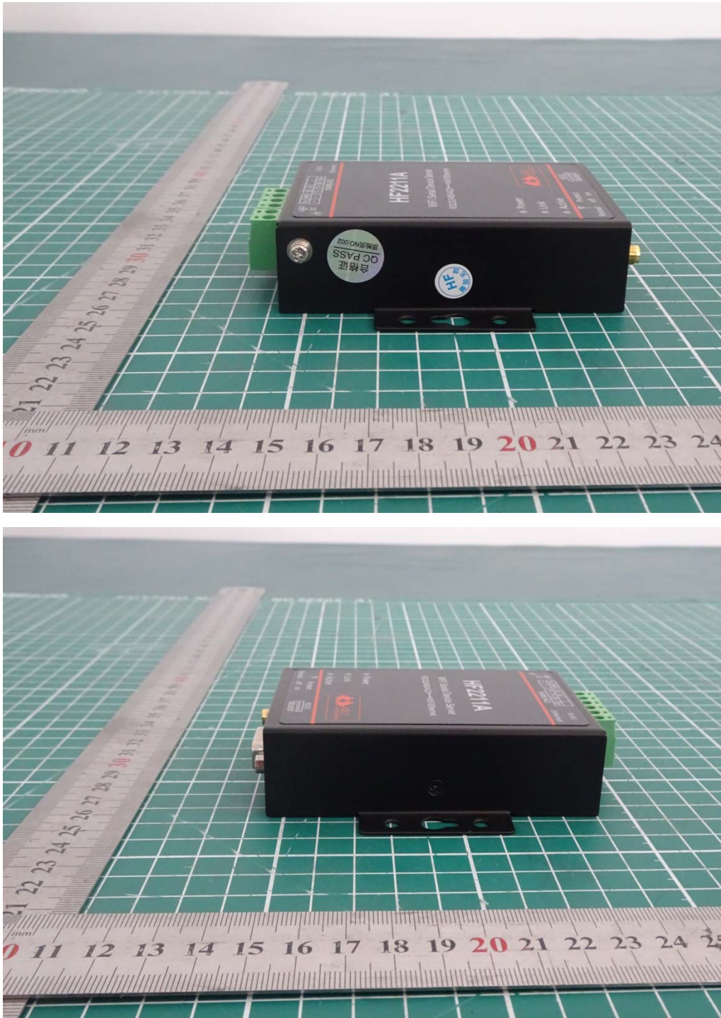
a: EUT
