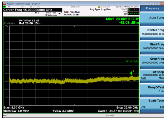
2480MHz,Plot 5,5000MHz~25000MHz
