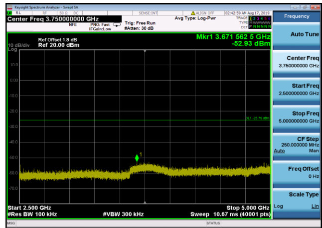
2480MHz,Plot 4,2500MHz~5000MHz
