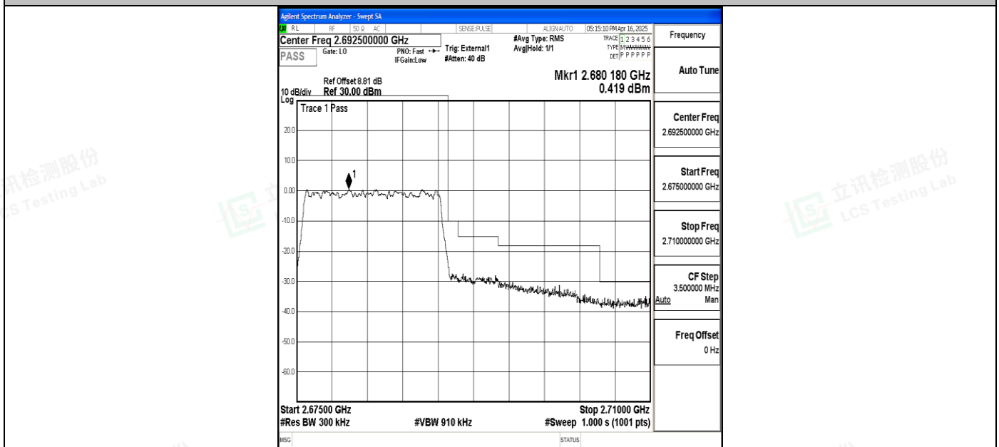
Band41_15MHz_QPSK_41515_75RB#0
