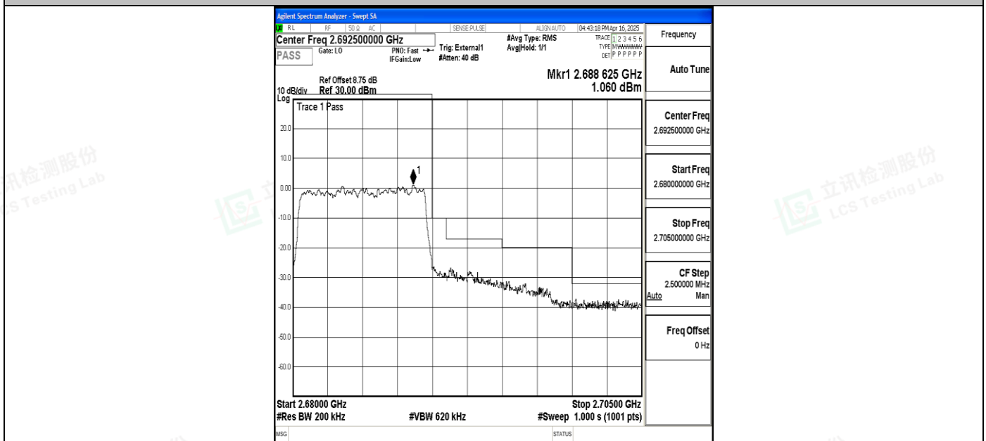
Band41_10MHz_QPSK_41540_50RB#0
