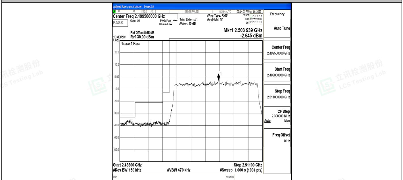
Band41_15MHz_QPSK_39725_75RB#0
