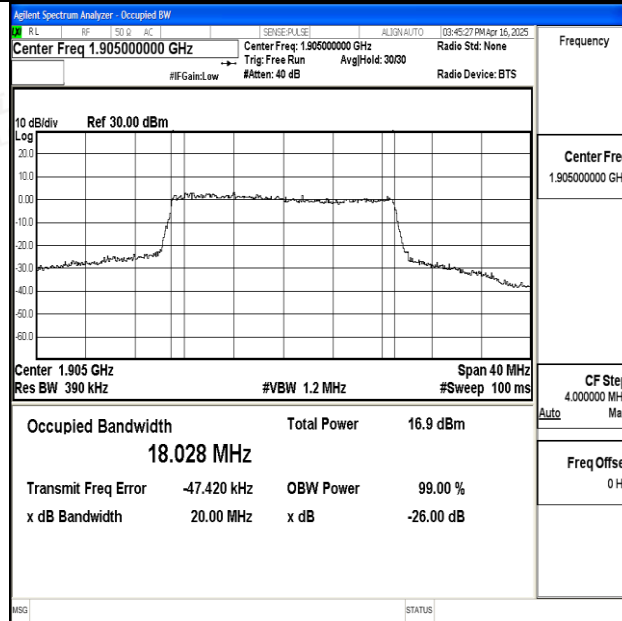
Band25-20MHz-QPSK-26590-100RB#0-PASS
