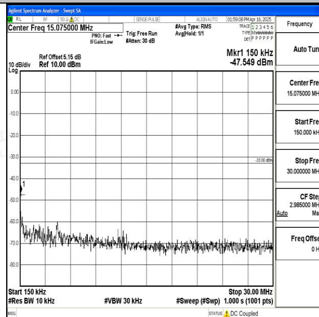
Band25 1.4MHz QPSK 26365 1RB#0 0.15~30 0.15~30
