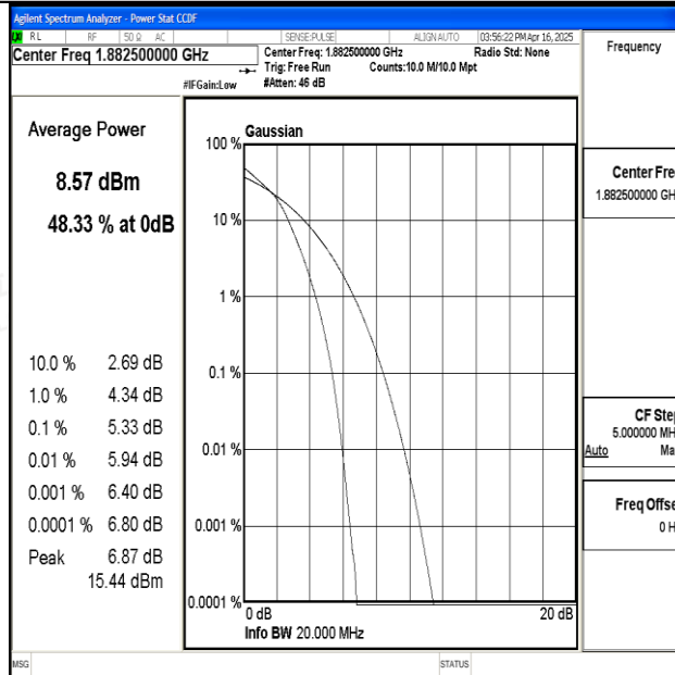
Band25-20MHz-16QAM-26365-100RB#0-PASS
