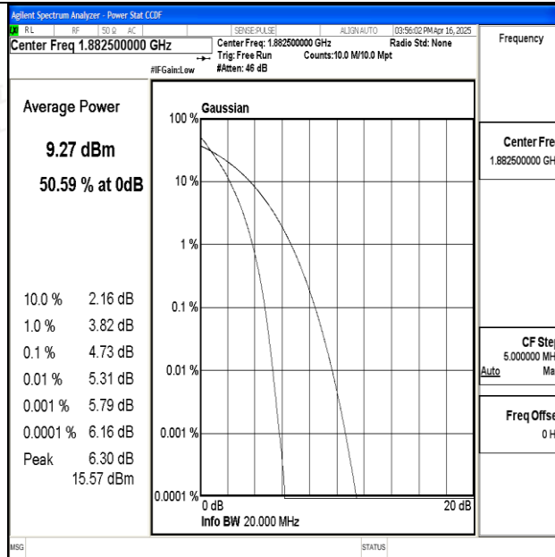
Band25-20MHz-QPSK-26365-100RB#0-PASS
