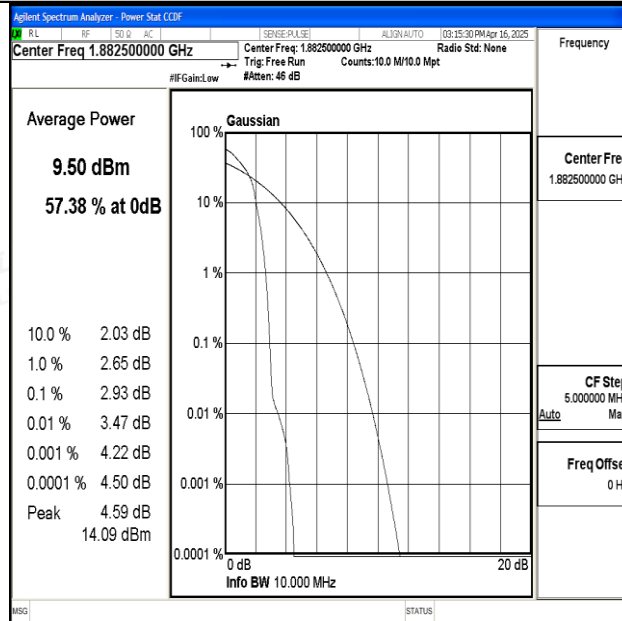
Band25-10MHz-16QAM-26365-1RB#0-PASS
