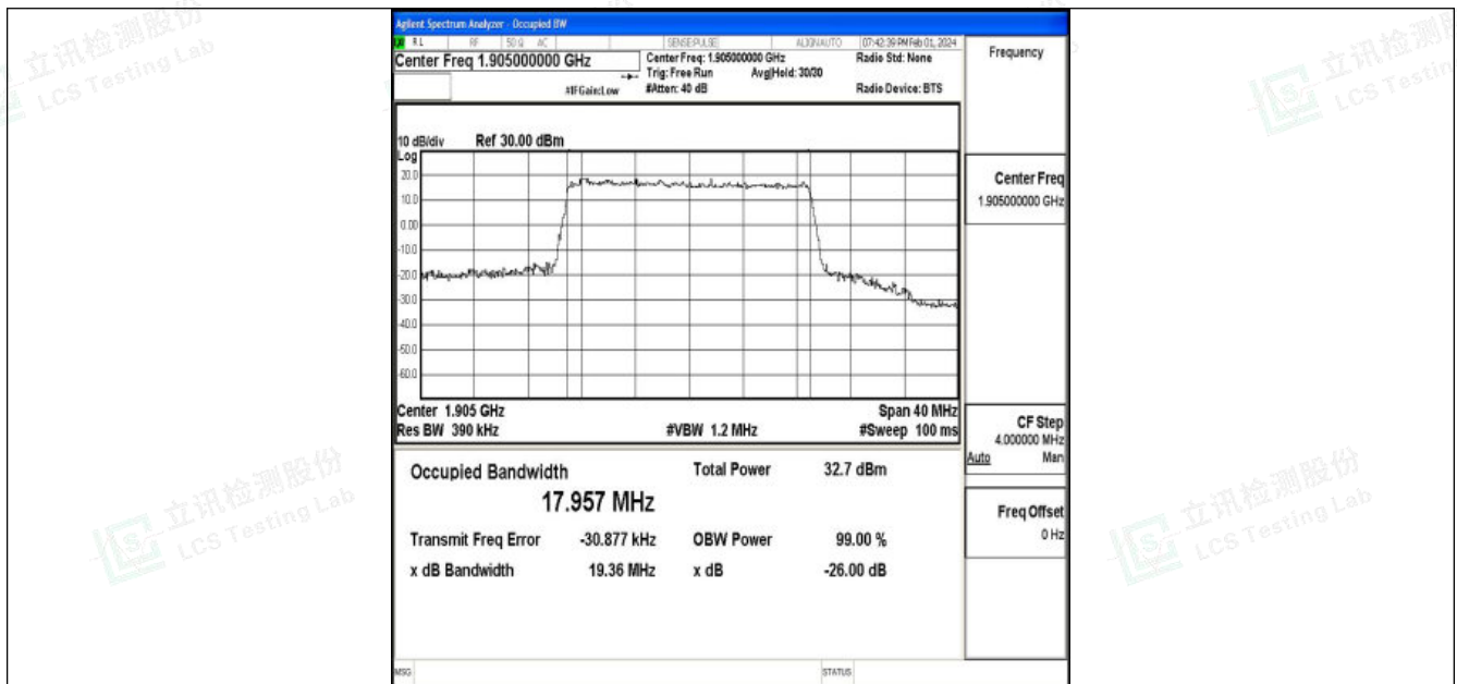
Band25-20MHz-QPSK-26590-100RB#0-PASS
