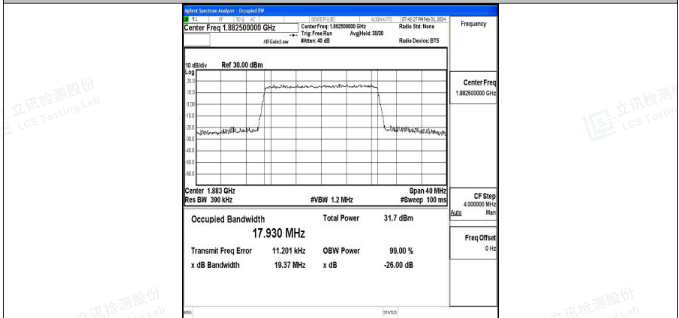
Band25-20MHz-16QAM-26365-100RB#0-PASS
