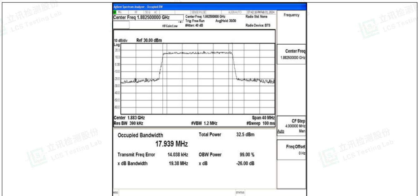
Band25-20MHz-QPSK-26365-100RB#0-PASS
