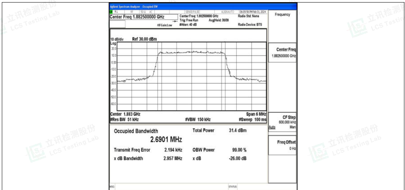
Band25-3MHz-QPSK-26365-15RB#0-PASS
