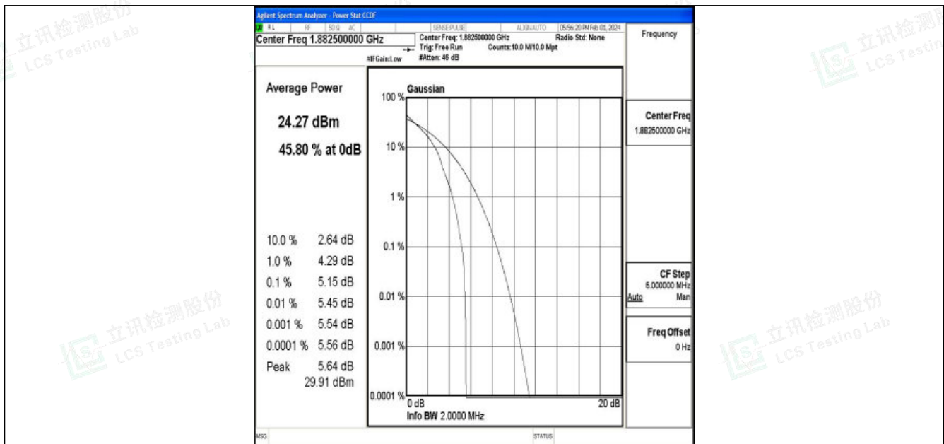
Band25-1.4MHz-QPSK-26365-1RB#0-PASS
