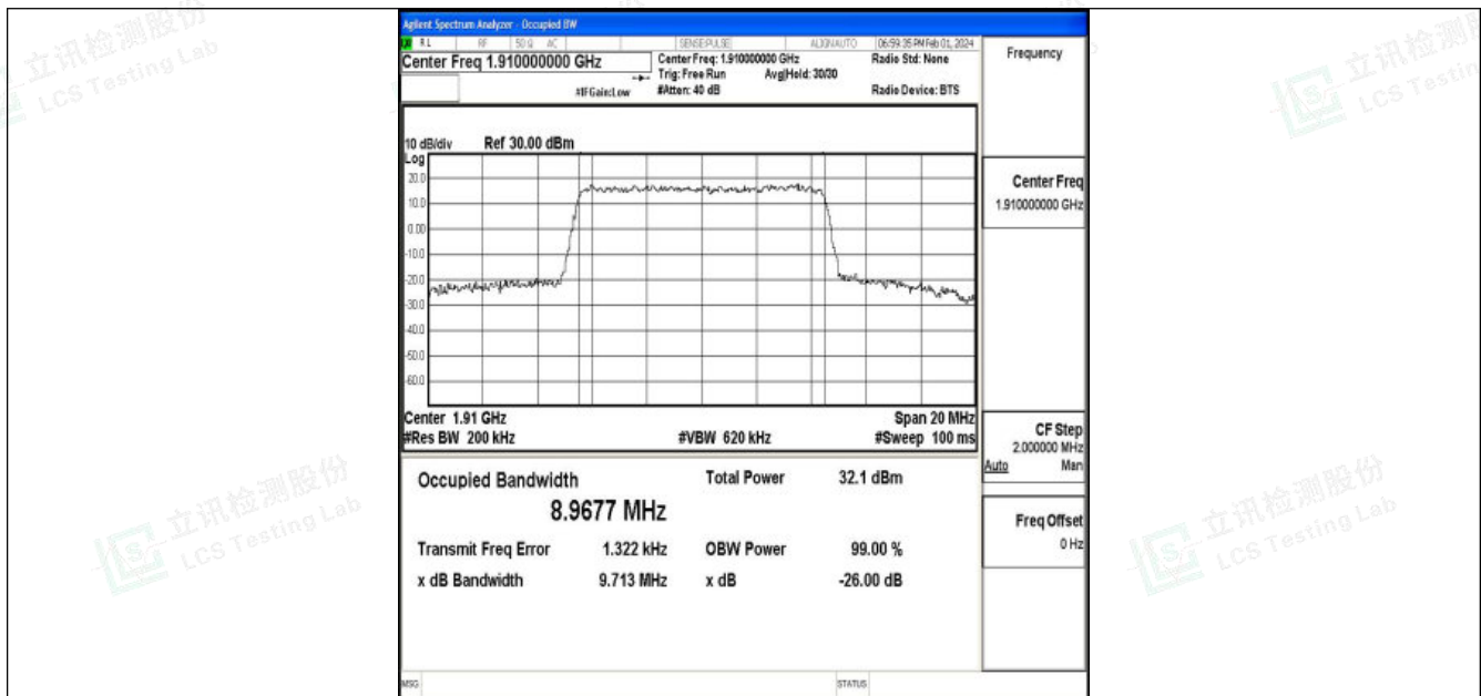
Band25-10MHz-QPSK-26640-50RB#0-PASS
