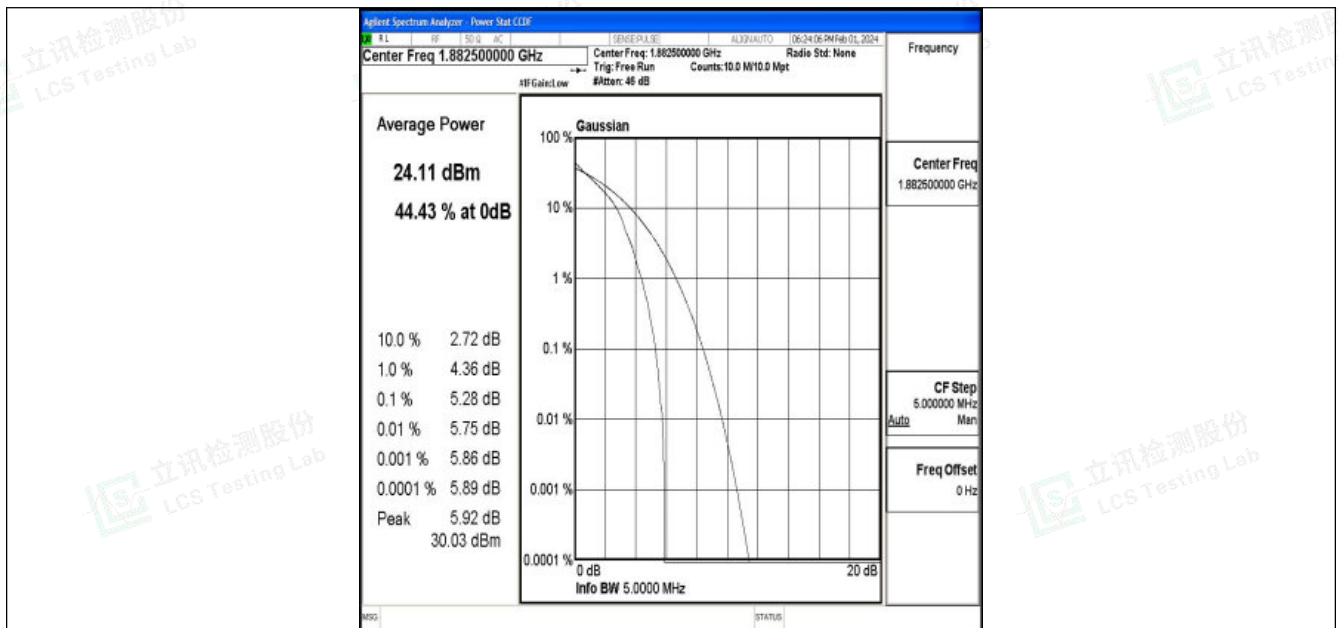
Band25-3MHz-QPSK-26365-1RB#0-PASS
