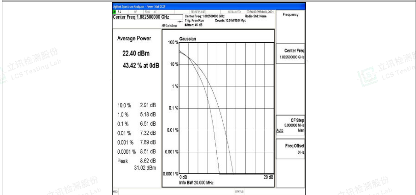
Band25-20MHz-16QAM-26365-100RB#0-PASS
