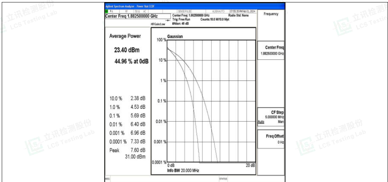
Band25-20MHz-QPSK-26365-100RB#0-PASS
