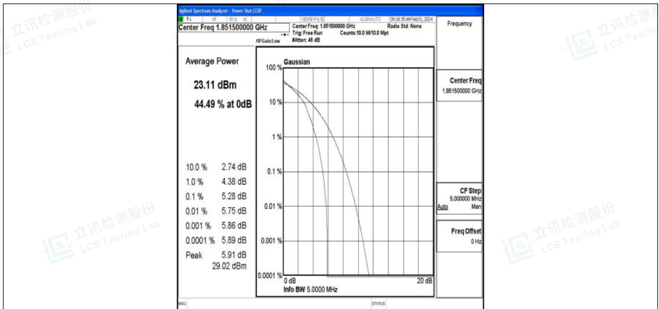
Band2-3MHz-QPSK-18615-1RB#0-PASS
