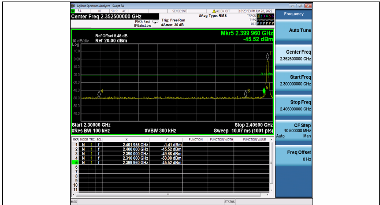
BLE 1M Ant1 Low 2402
