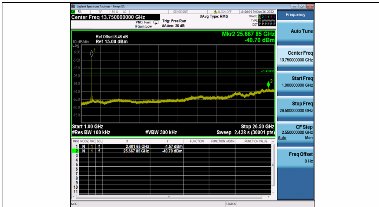
BLE 1M Ant1 2402 1000~26500
