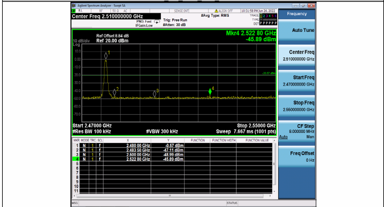
BLE 1M Ant1 High 2480
