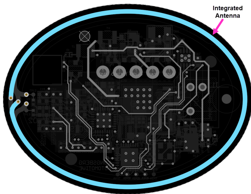
Inner Layer 2
