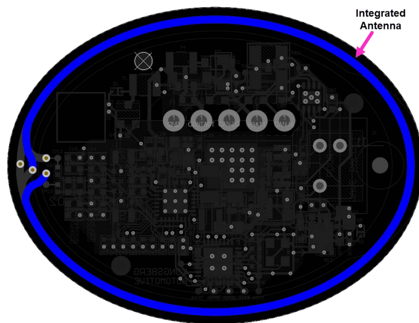
Bottom Layer
