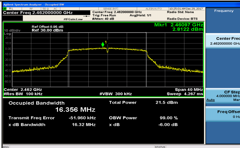
6dB Bandwidth_11G_2462_Ant1
