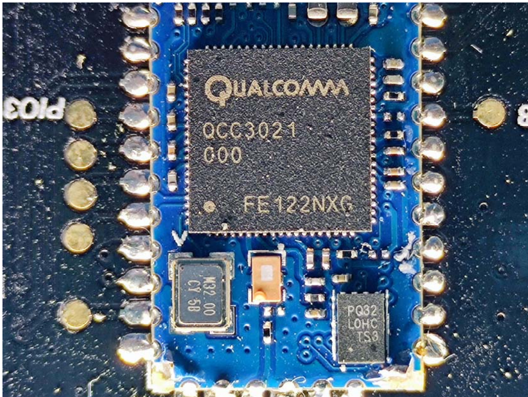
EUT Chip
