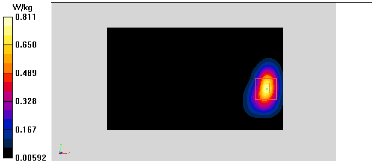
Fig.18 LTE Band4
