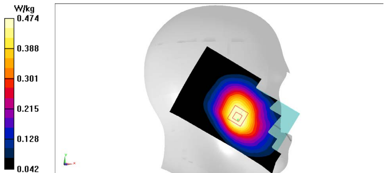
Fig.13 LTE Band5
