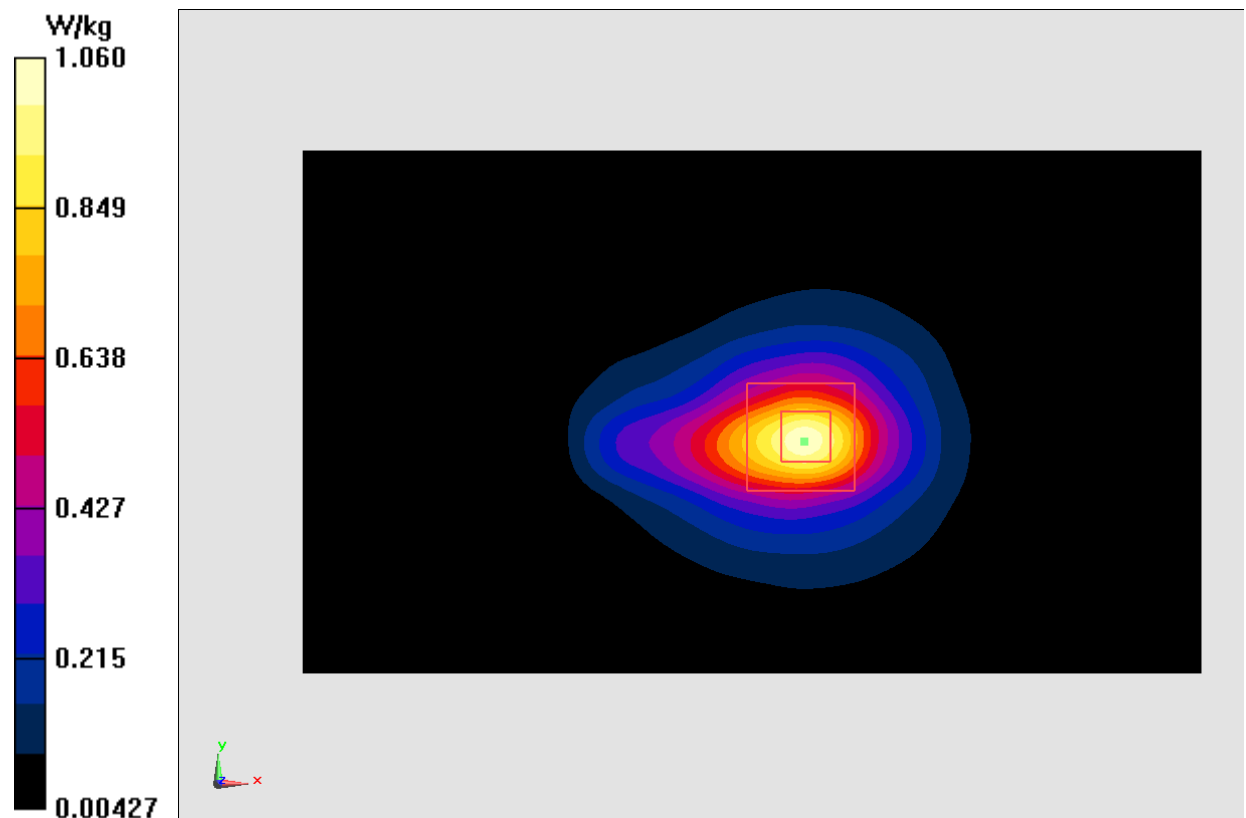
Fig.16 LTE Band7
