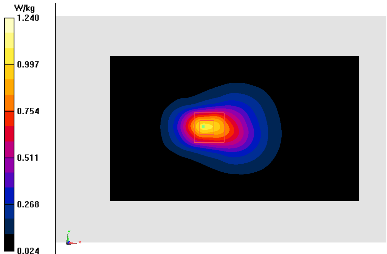
Fig.12 LTE Band4
