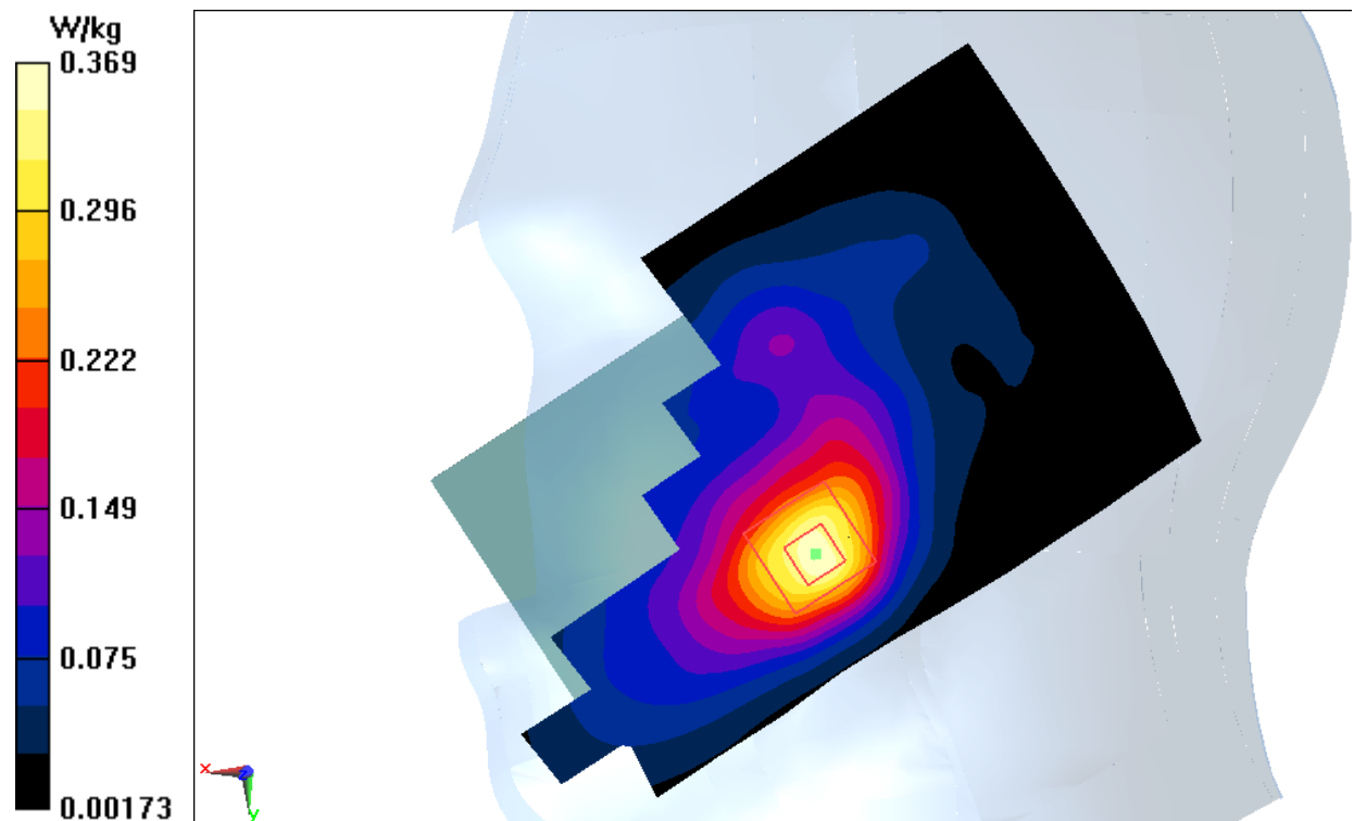
Fig.15 LTE Band7
