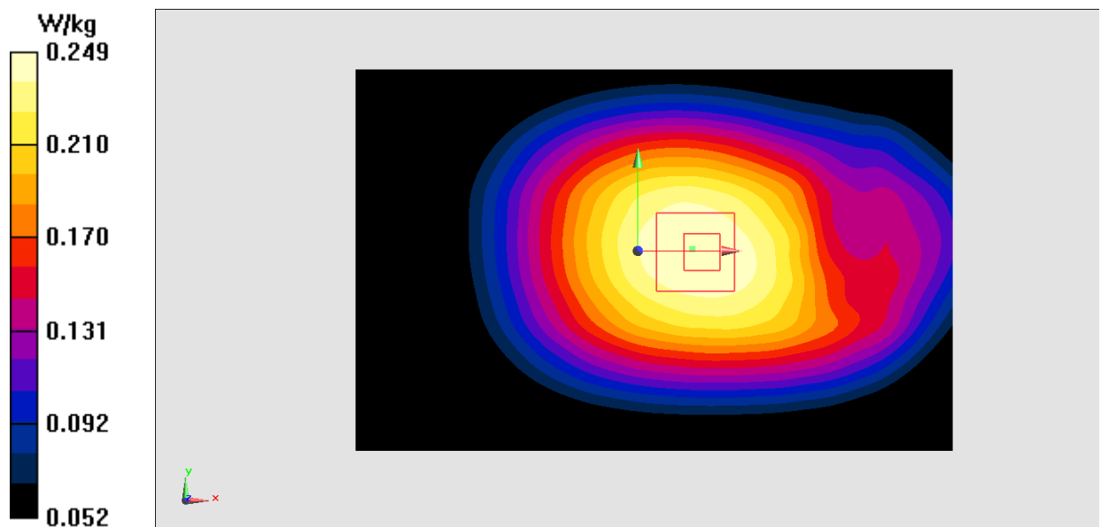
Fig.20 LTE Band13
