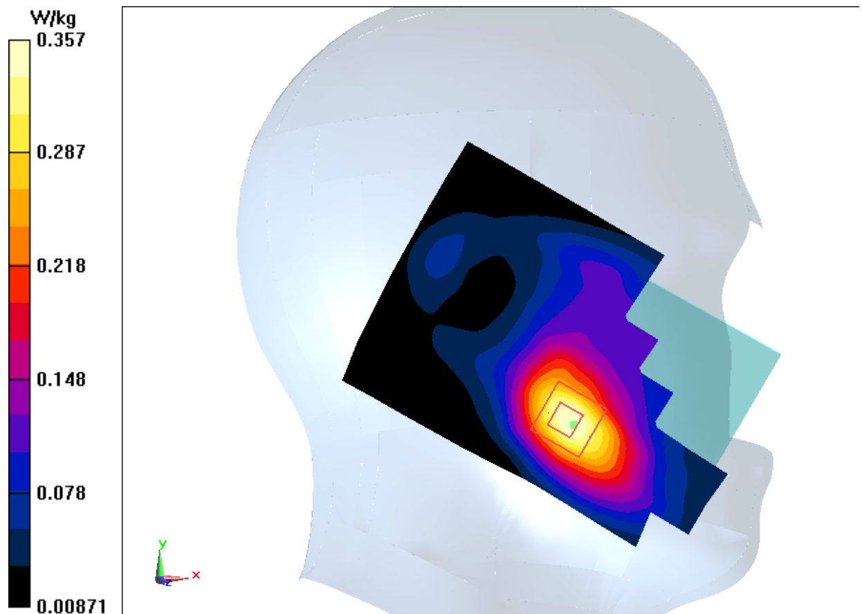
Fig.7 1700MHz
