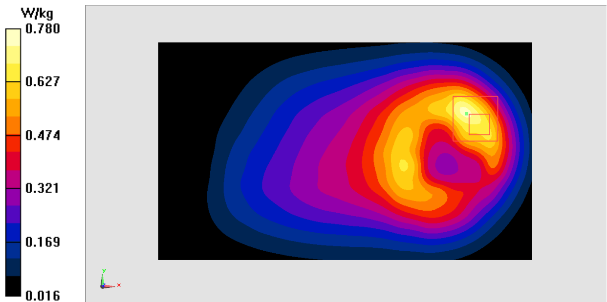
Fig.16 LTE Band5
