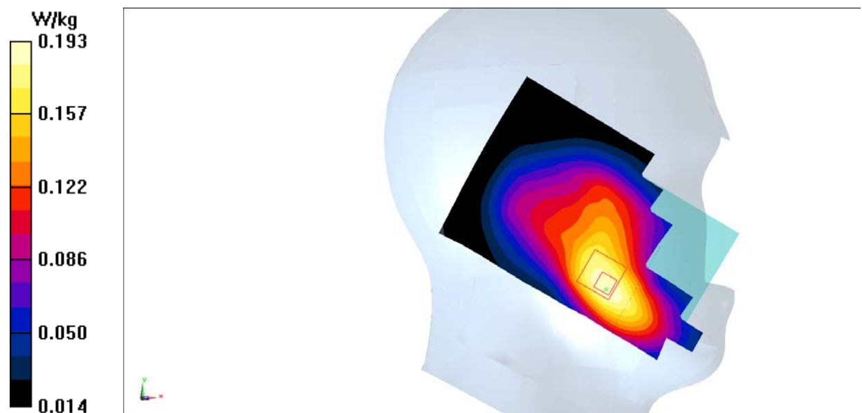
Fig.19 LTE Band17
