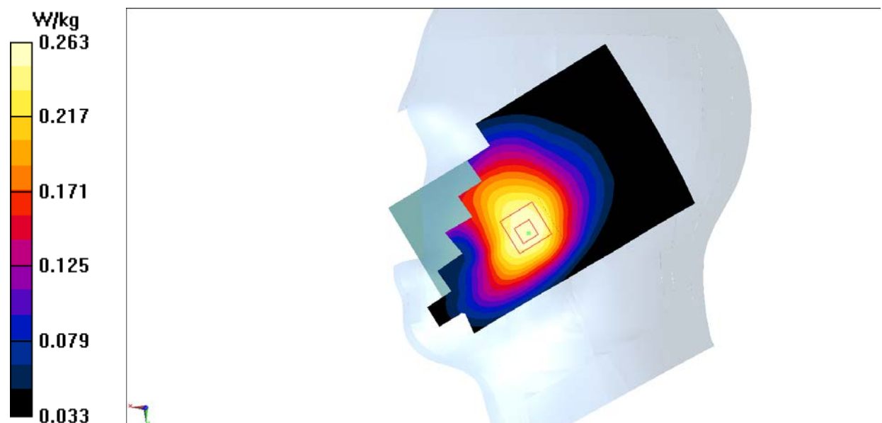
Fig.5 WCDMA 850
