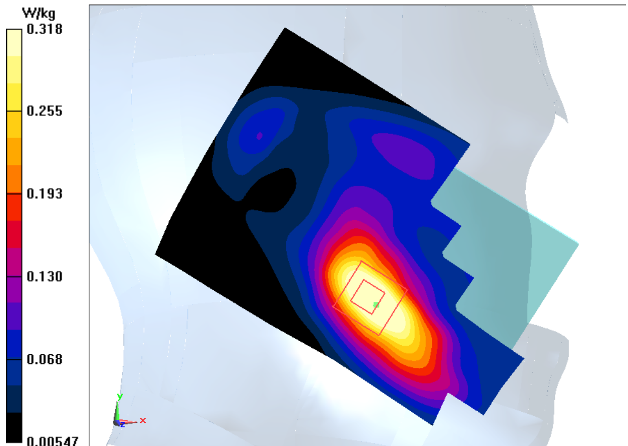
Fig.9 WCDMA1900
