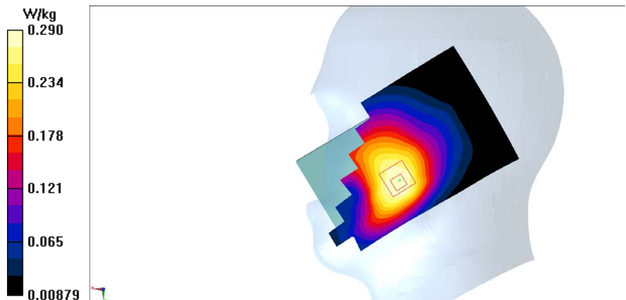
Fig.15 LTE Band5
