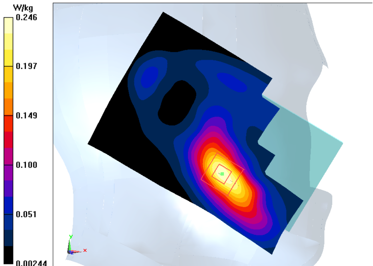
Fig.11 LTE Band2
