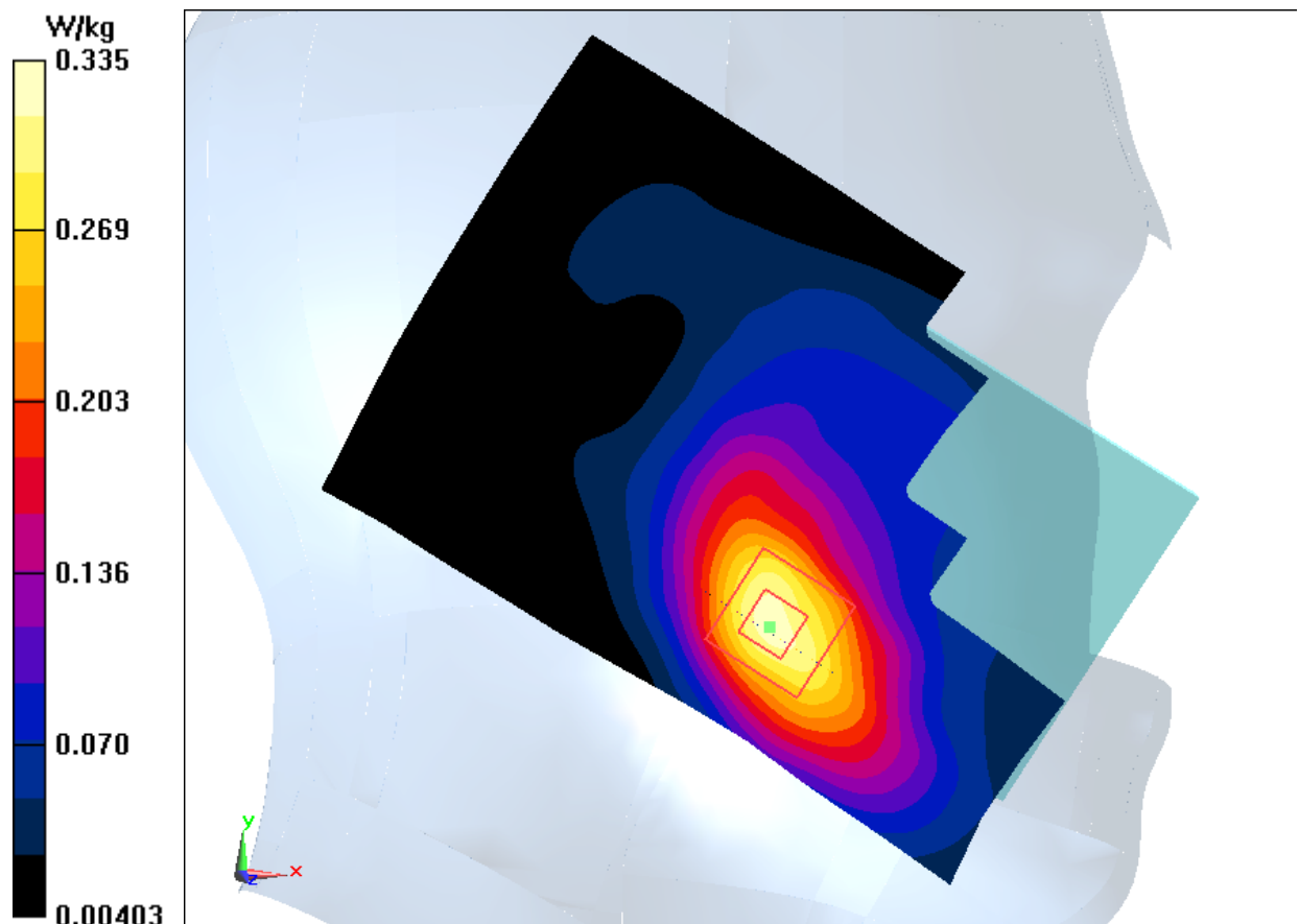
Fig.13 LTE Band4
