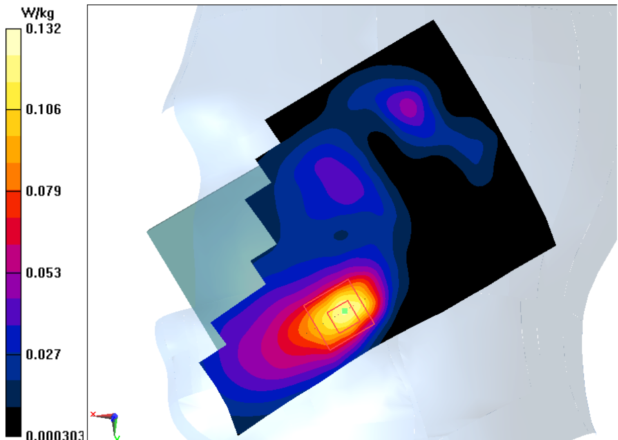
Fig.17 LTE Band7
