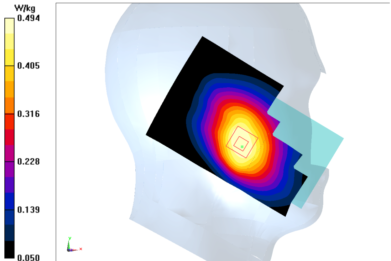
Fig.19 LTE Band5
