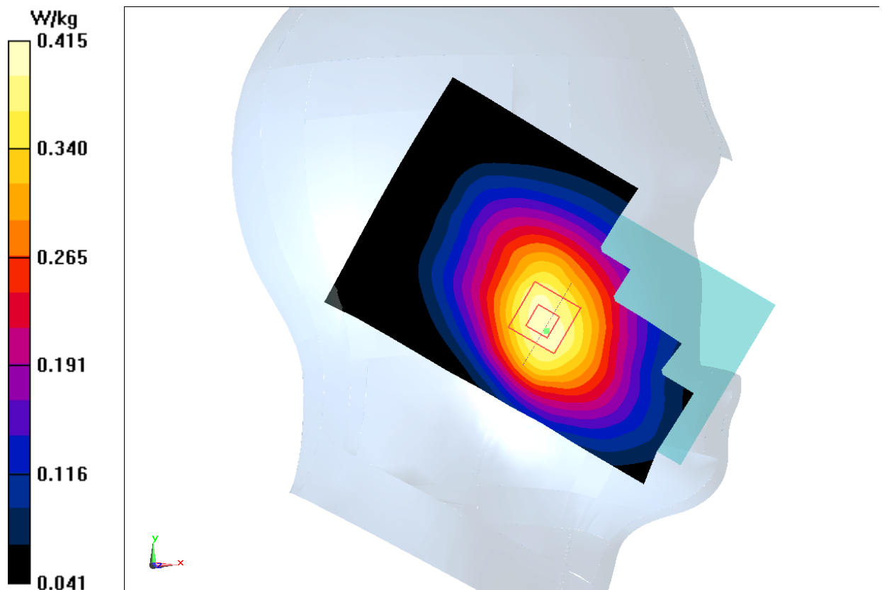
Fig.21 LTE Band5
