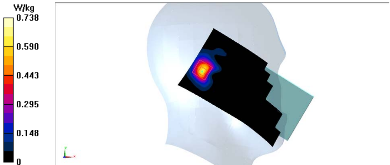
Fig.25 5GHz
