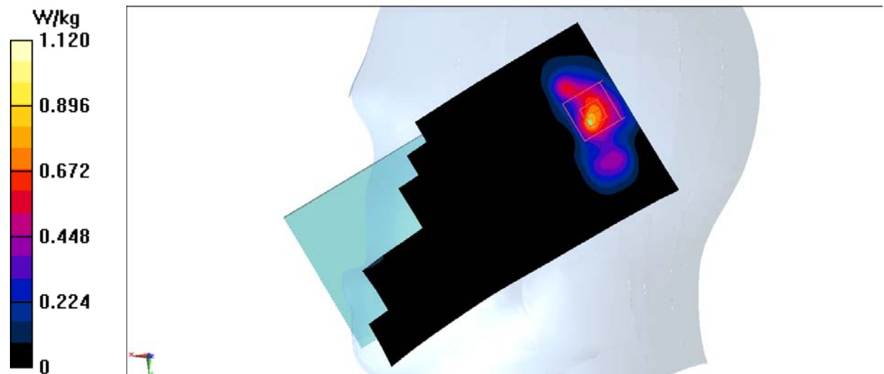
Fig.27 5GHz
