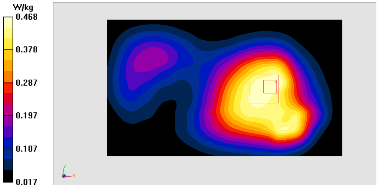
Fig.12 LTE Band4
