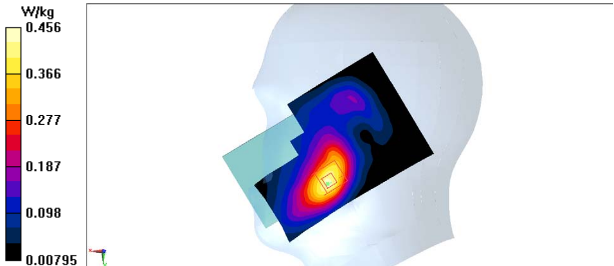
Fig.17 1700MHz
