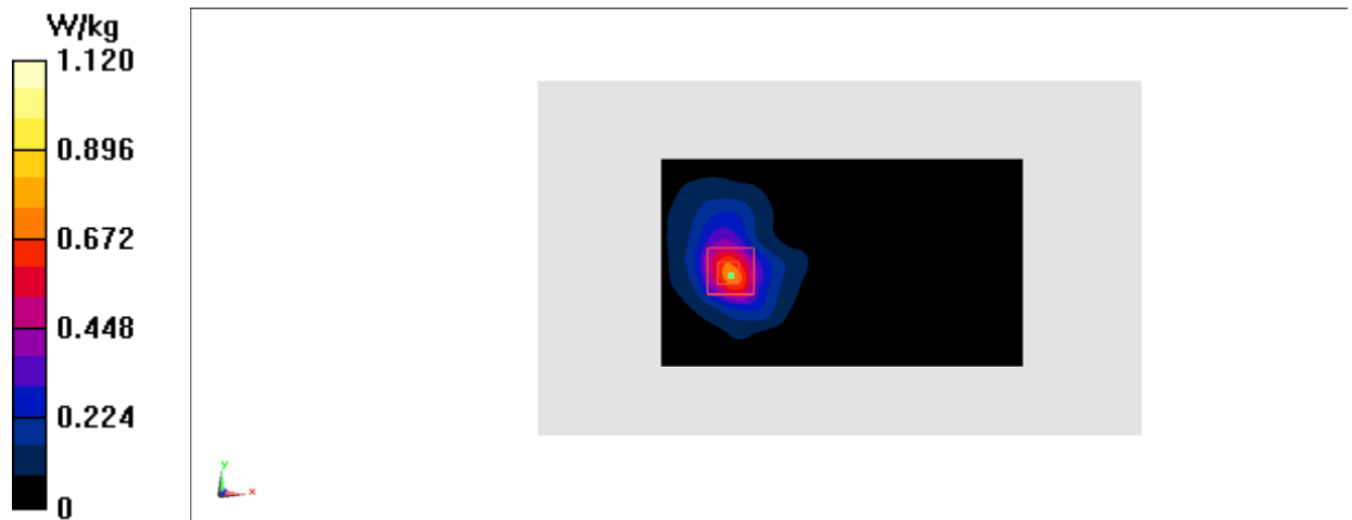
Fig.24 5GHz
