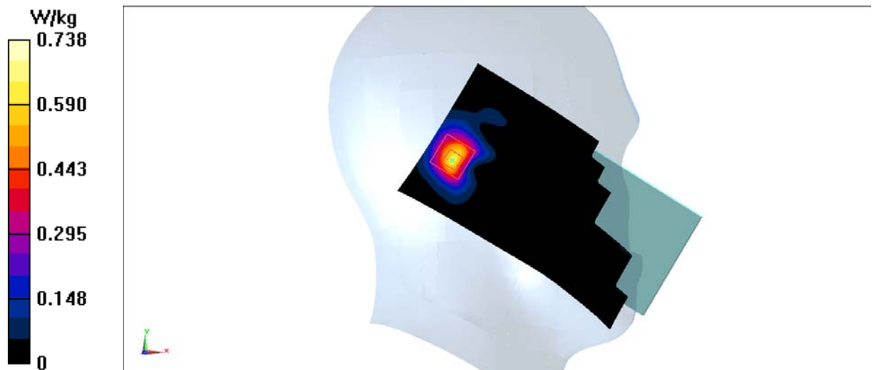
Fig.21 5GHz
