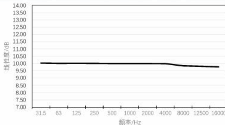
图 2 HATS 右耳线性度图
