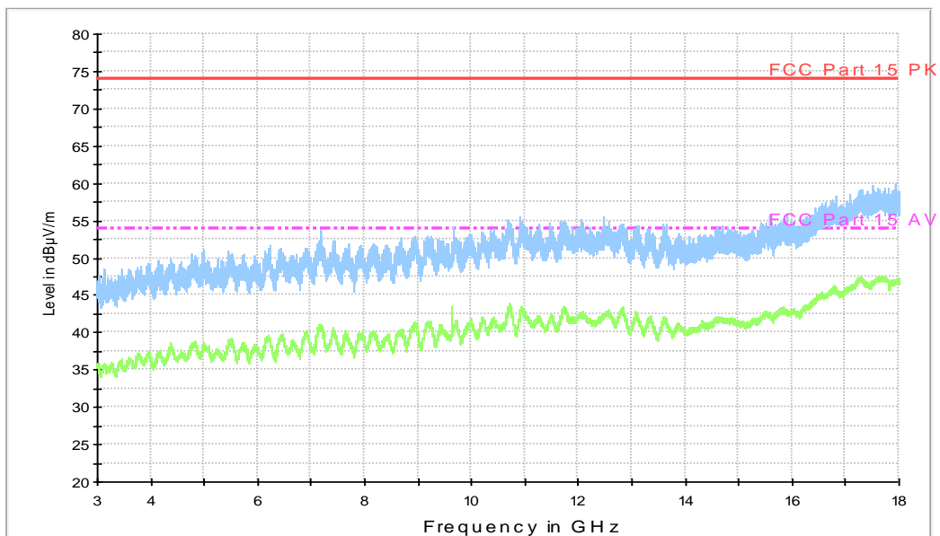
RE - 3GHz-18GHz
