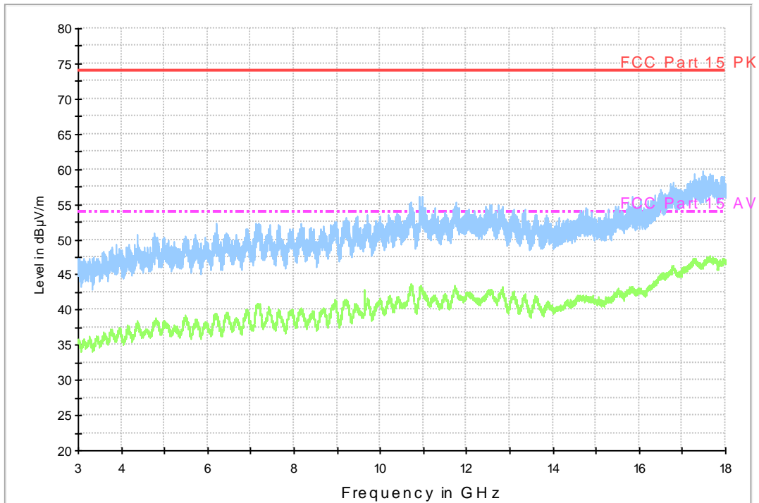
RE - 3GHz-18GHz
