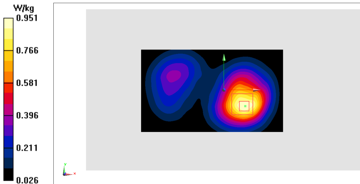
Fig.10 WCDMA1900
