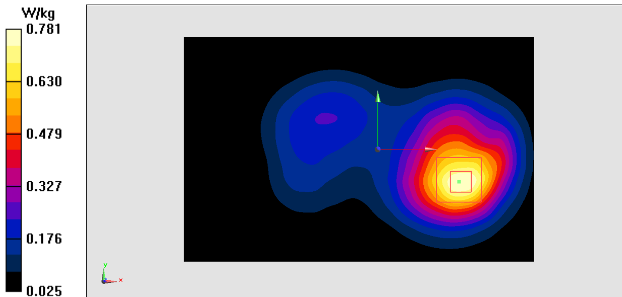
Fig.12 LTE Band2
