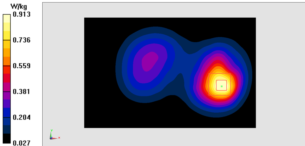
Fig.14 LTE Band4
