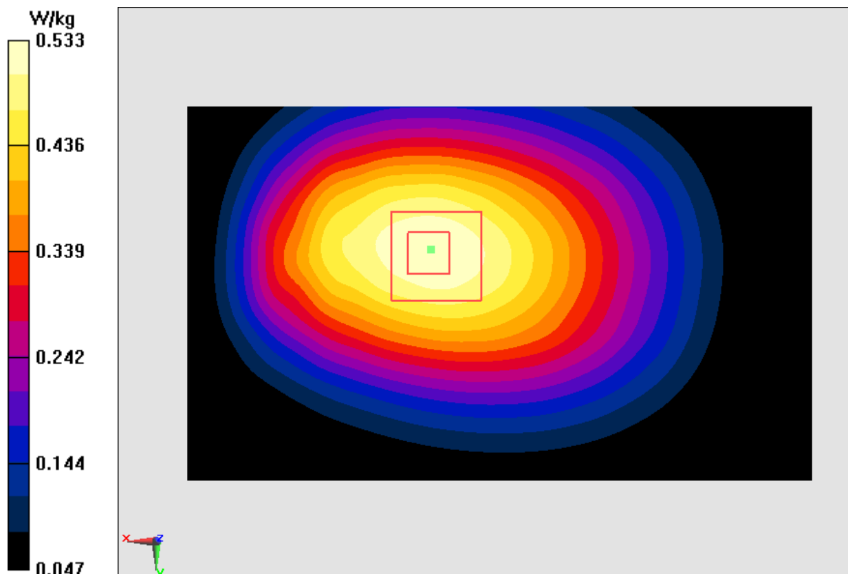
Fig.20 LTE Band13
