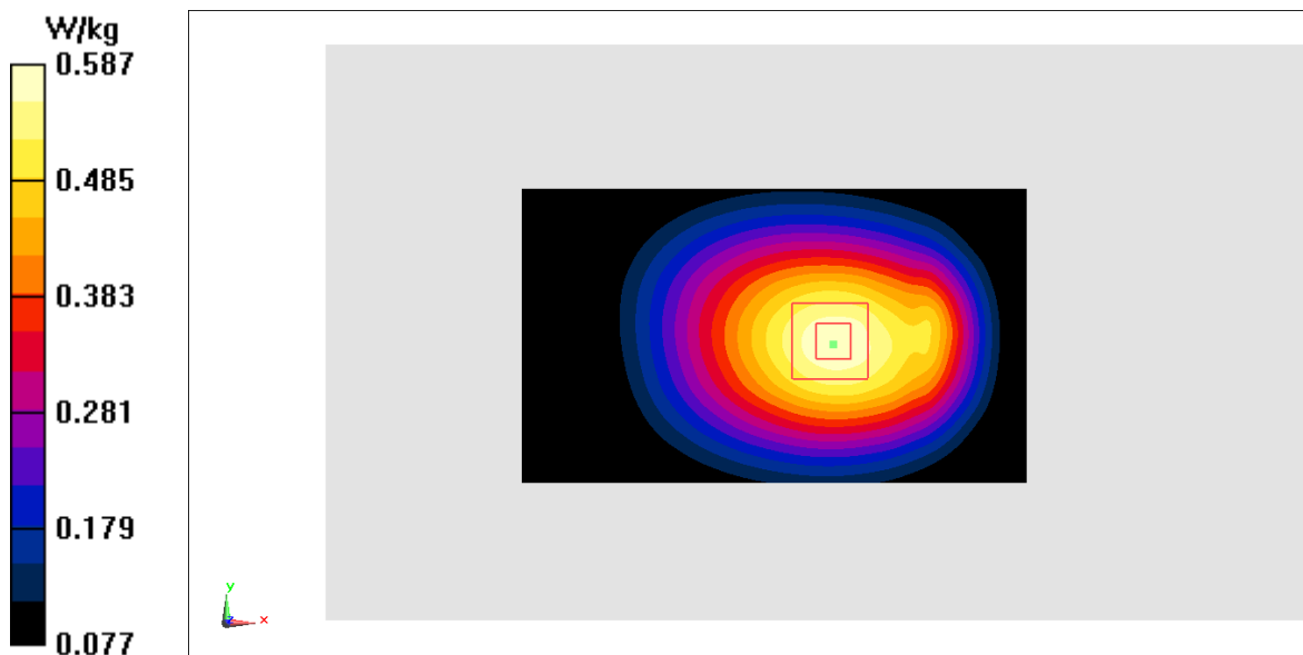
Fig.6 WCDMA 850
