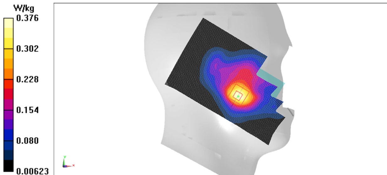
Fig.11 LTE Band2
