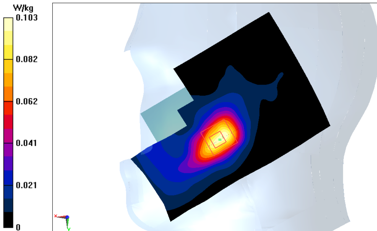
Fig.15 LTE Band7
