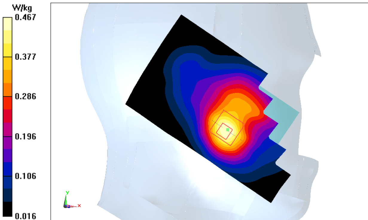
Fig.7 WCDMA1700
