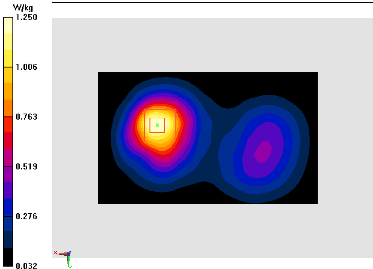
Fig.8 WCDMA1700
