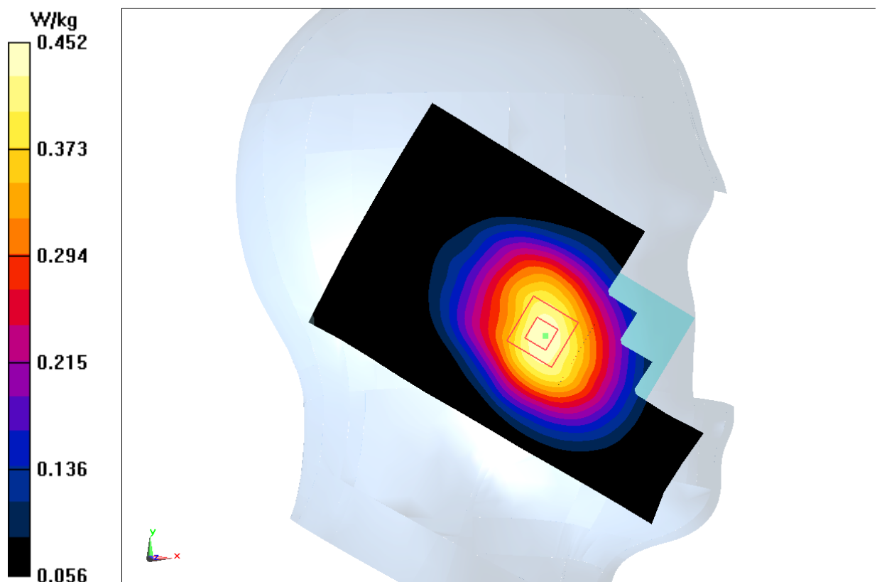
Fig.5 WCDMA 850
