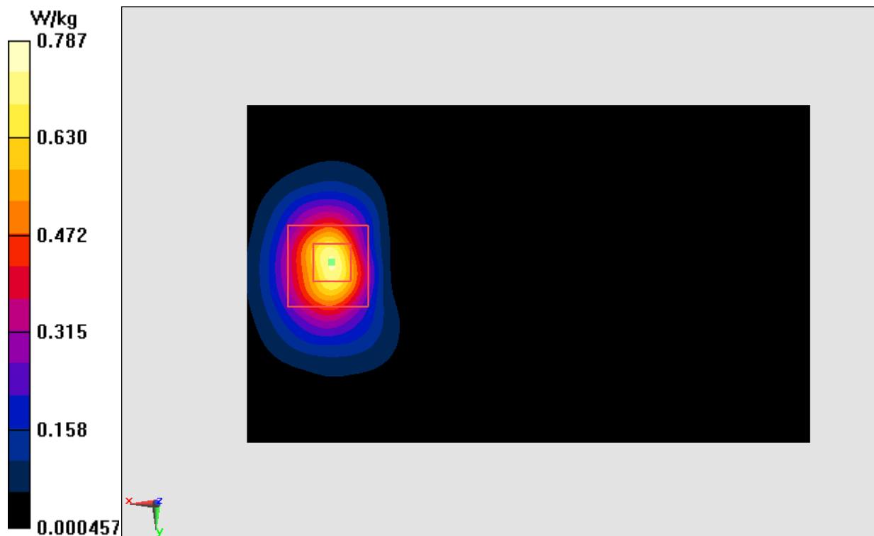
Fig.16 LTE Band7
