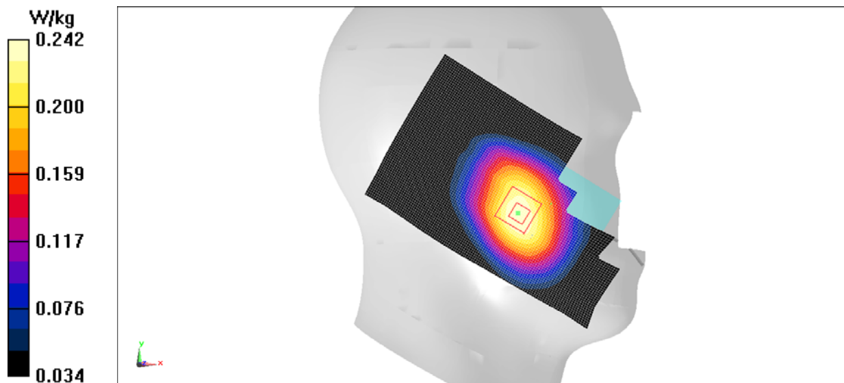
Fig.19 LTE Band13
