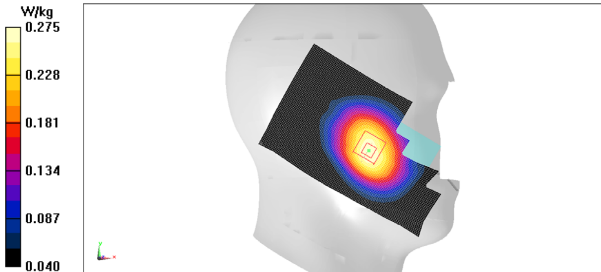
Fig.13 LTE Band4
