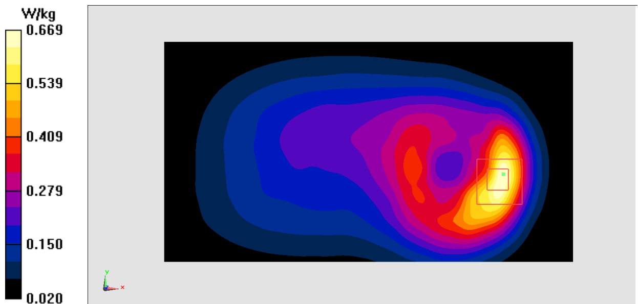
Fig.6 WCDMA 850
