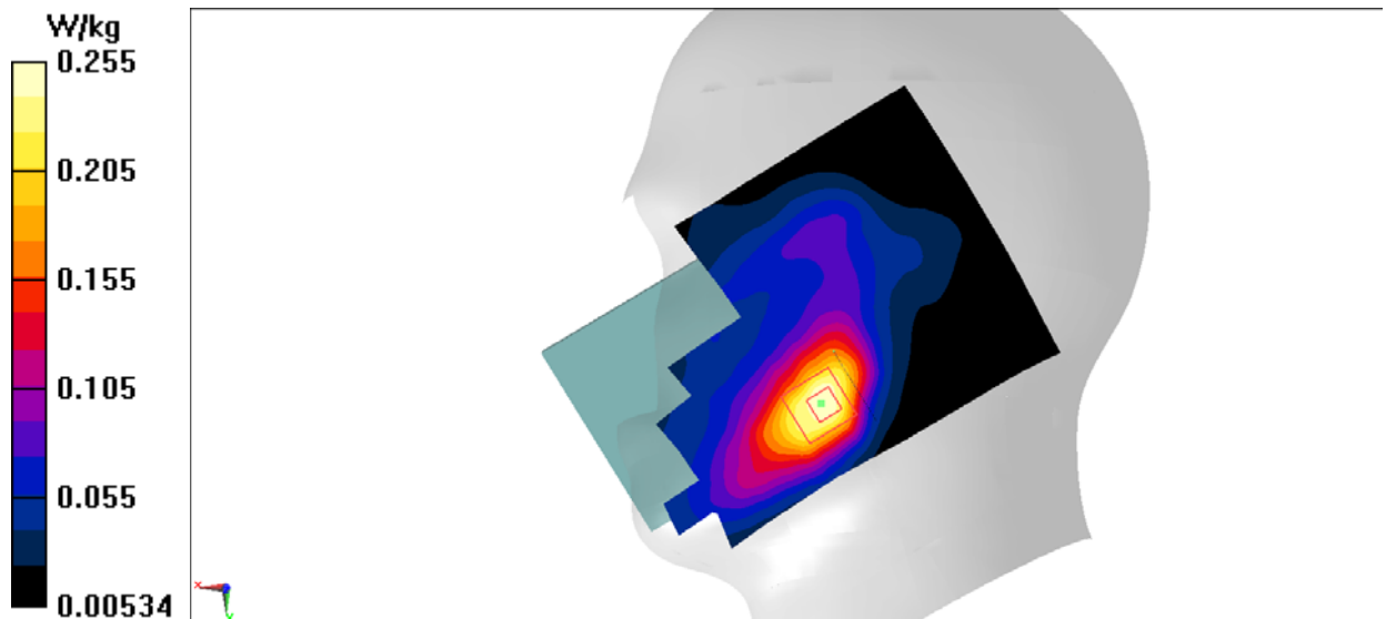
Fig.13 LTE Band4
