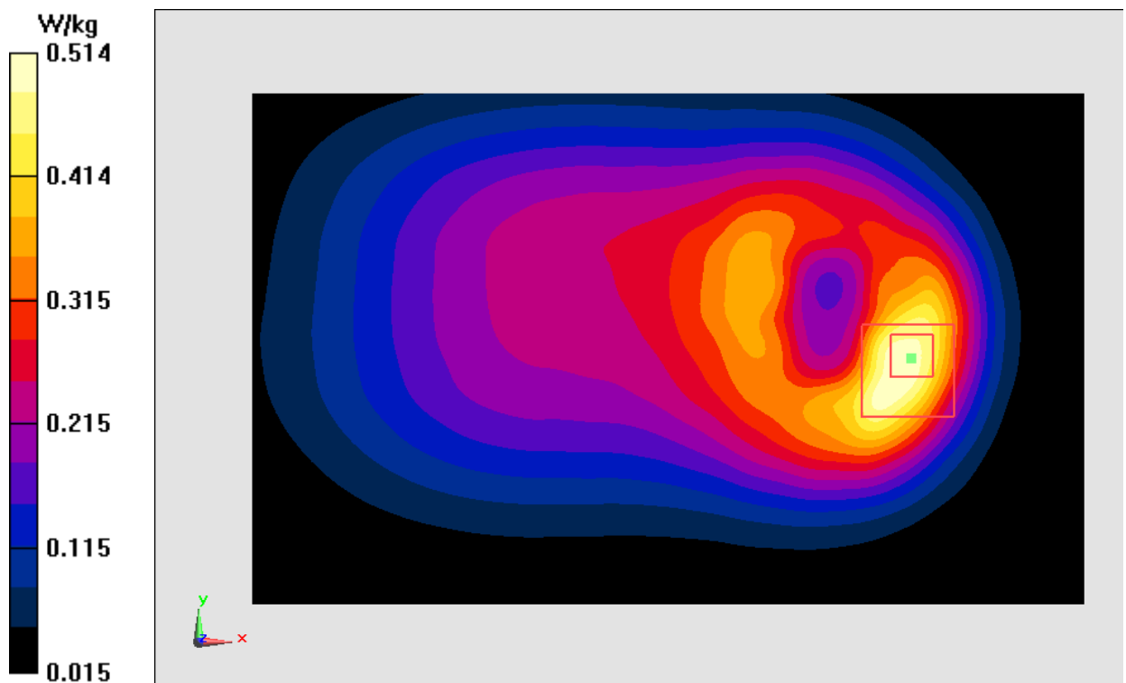
Fig.21 LTE Band13
