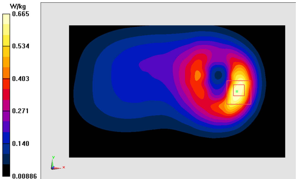
Fig.23 LTE Band5
