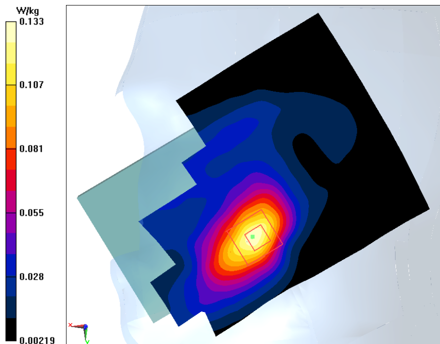
Fig.7 WCDMA1900
