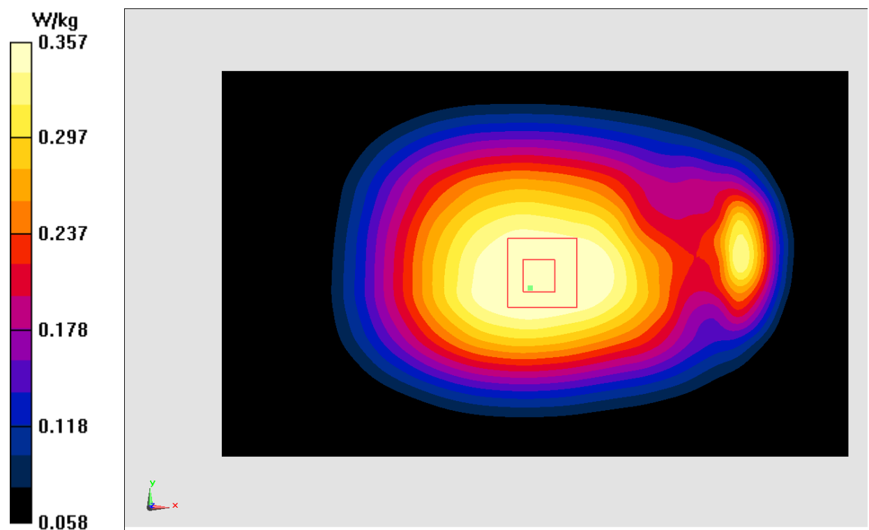
Fig.6 WCDMA 850
