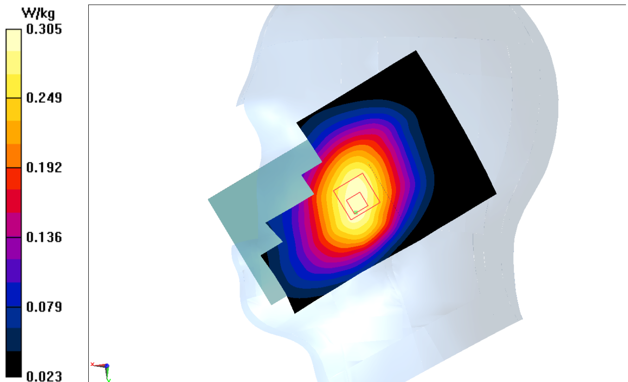
Fig.21 LTE Band5
