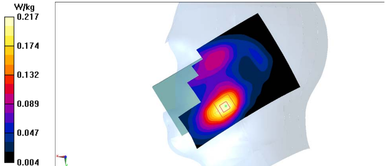
Fig.19 1700MHz
