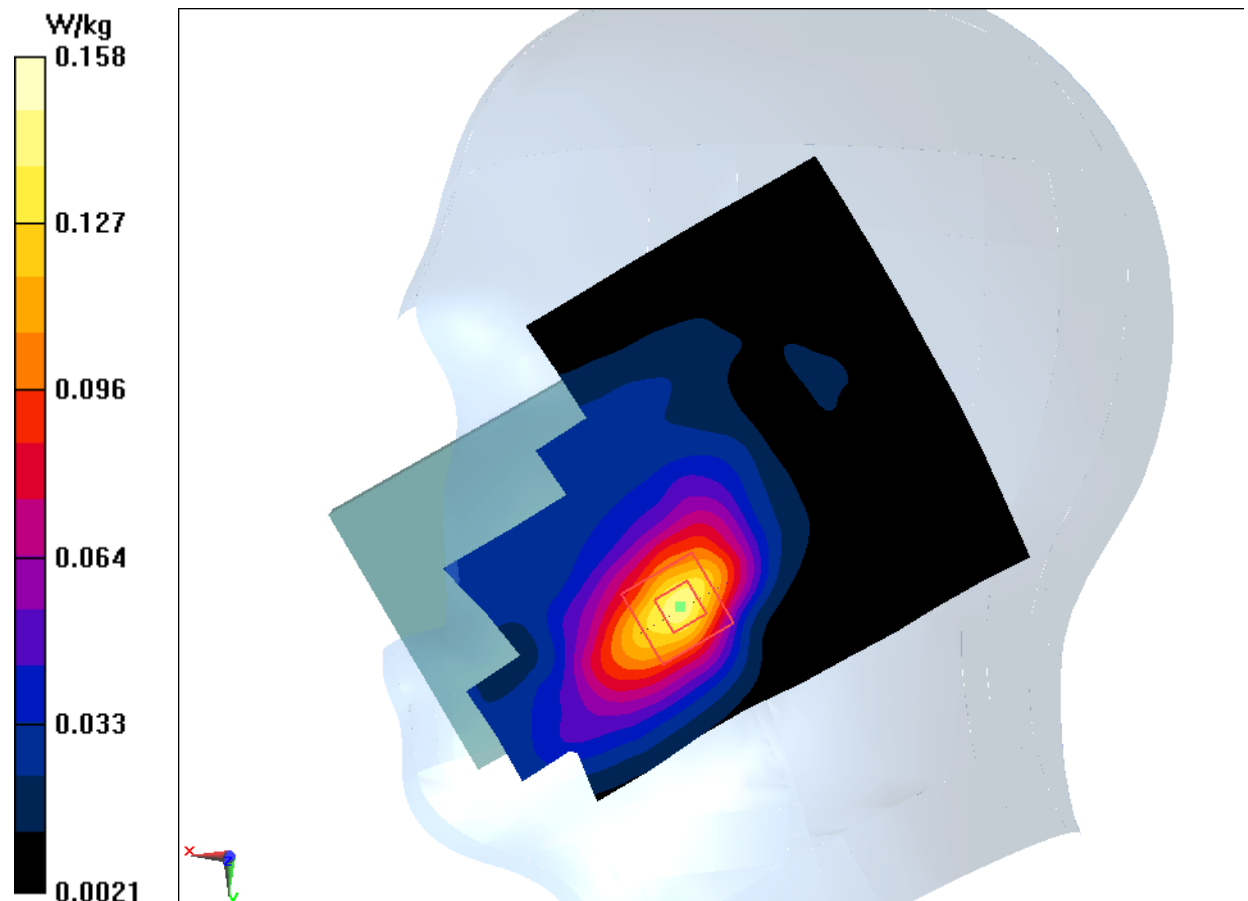
Fig.10 LTE Band2
