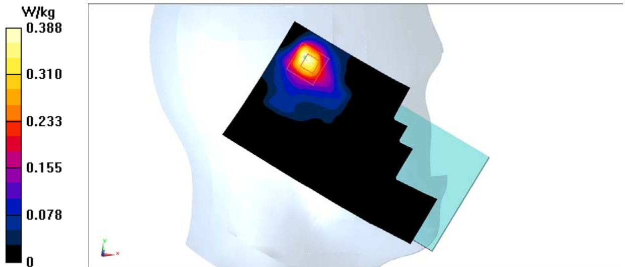
Fig.24 5GHz
