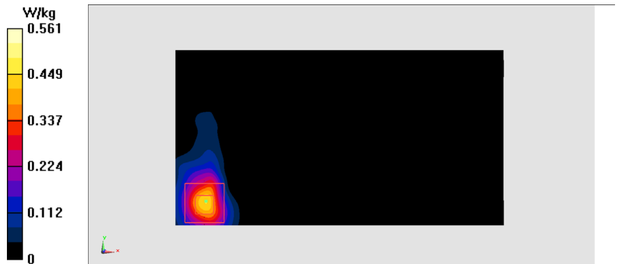
Fig.29 5GHz
