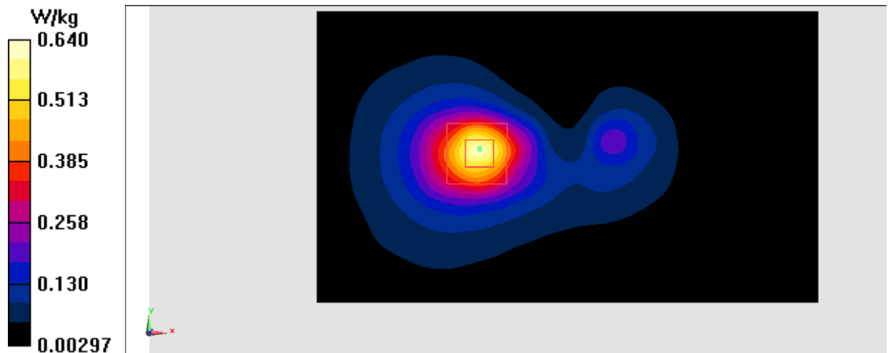
Fig.21 LTE Band30
