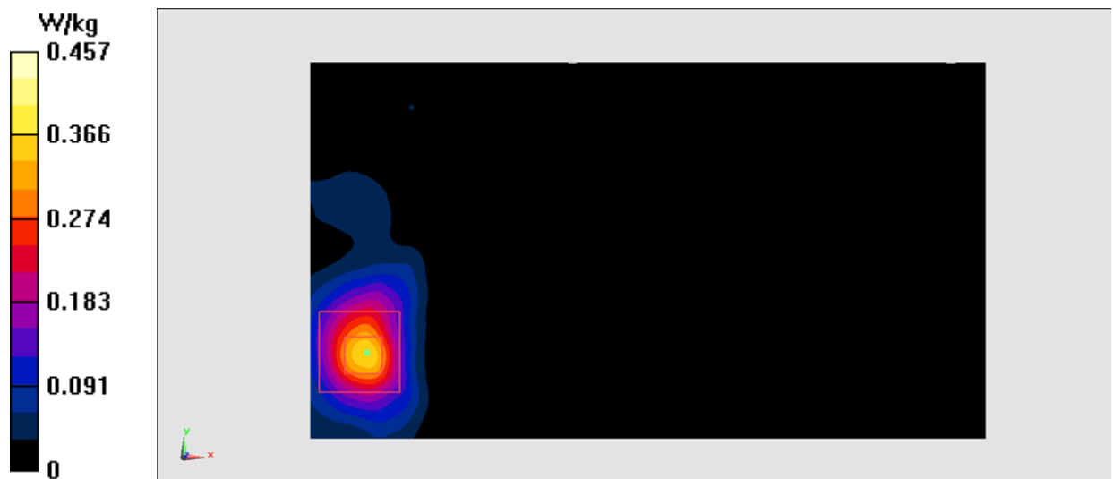
Fig.27 5GHz
