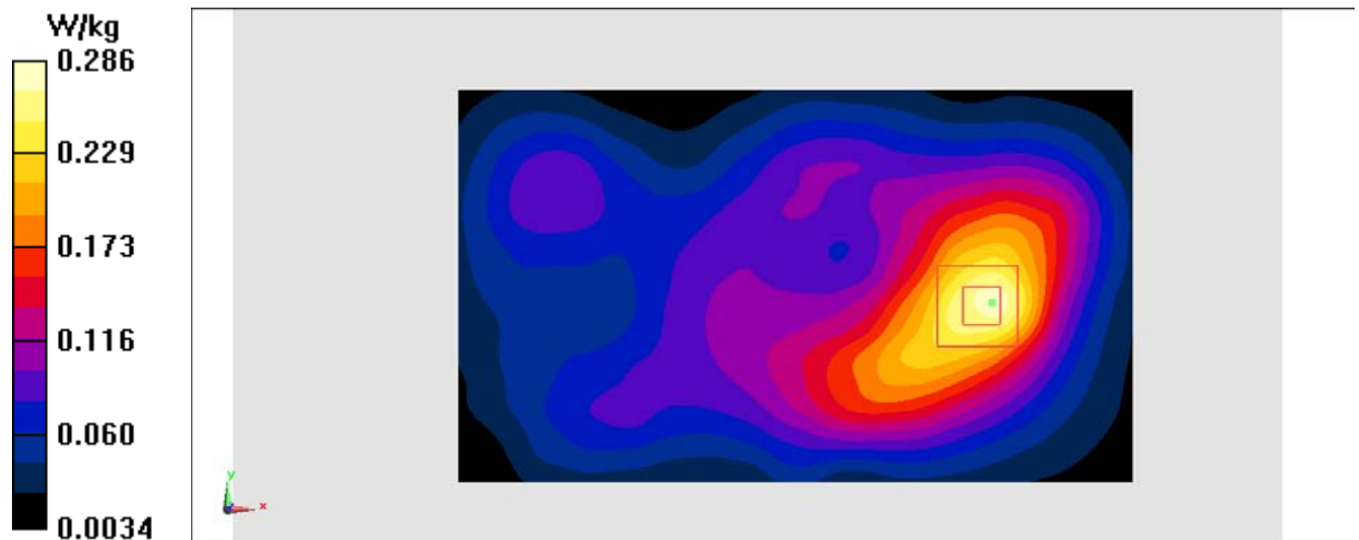
Fig.20 LTE Band30
