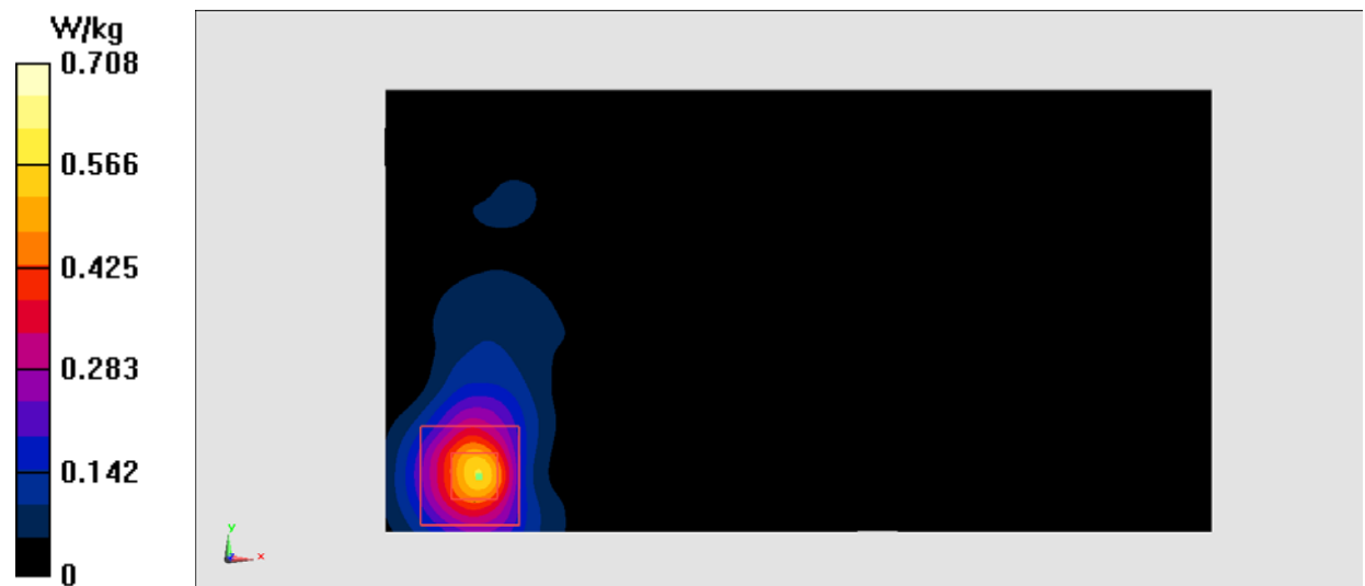
Fig.25 5GHz
