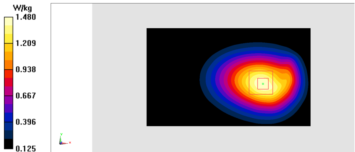
Fig.6 WCDMA 850
