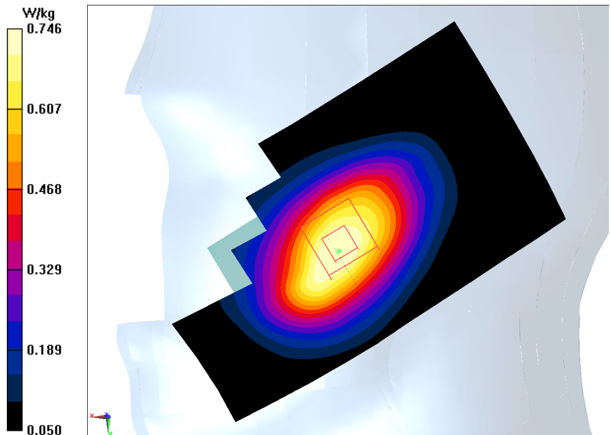
Fig.5 WCDMA 850
