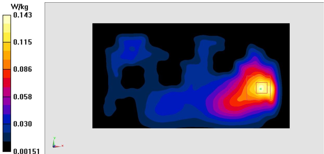
Fig.32 LTE Band30
