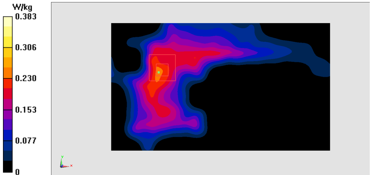
Fig.37 5GHz
