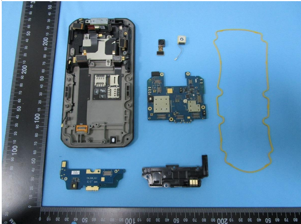
(2) EUT Photo
