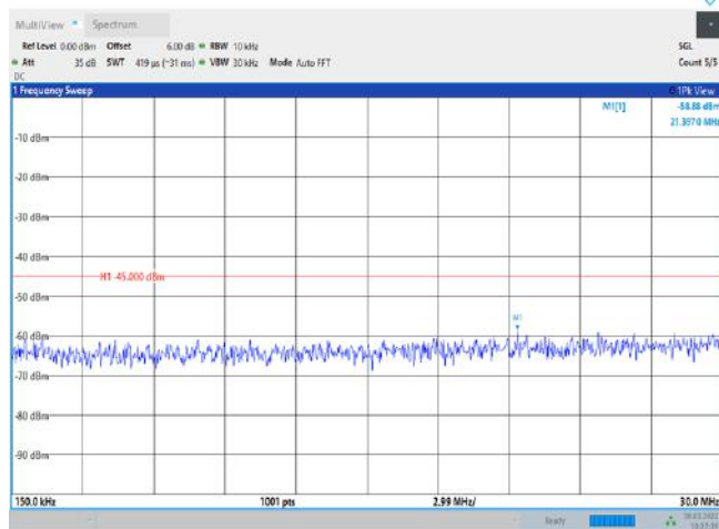
Band41-20MHz-QPSK-39750-1RB#0-Range2:0.15~30MHz
