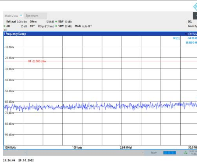
Band4-20MHz-QPSK-20050-1RB#0-Range2:0.15~30MHz
