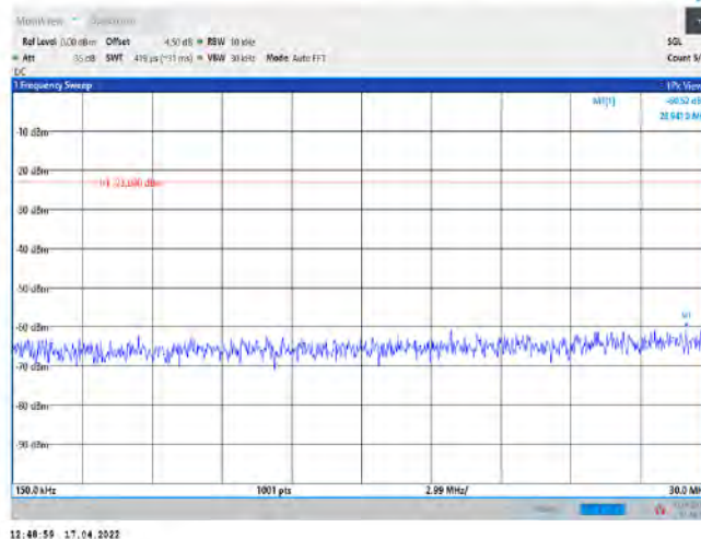
Band71-20MHz-QPSK-133222-1RB#0-Range2:0.15~30MHz
